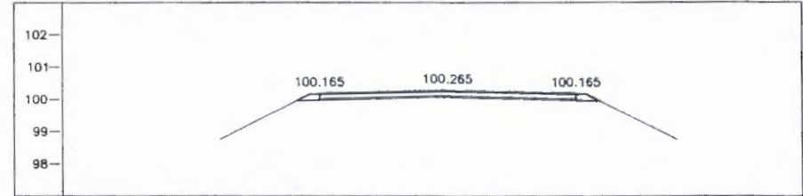
STA. 2+025.000 NGL = 99.934
