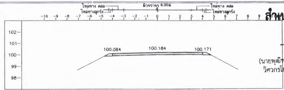
STA. 2+066.000 NGL = 100.034
