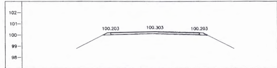
STA. 2+000.000 NGL = 99.931
