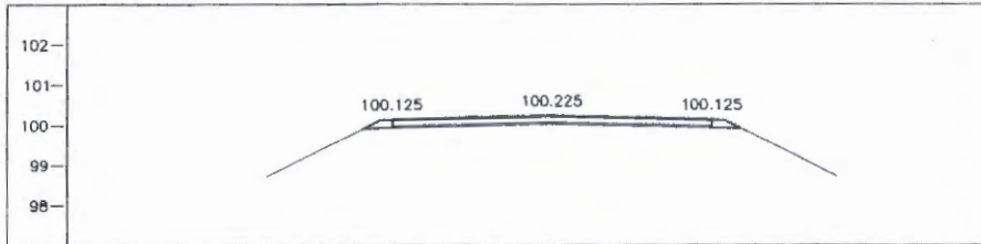
STA. 1+925.000 NGL = 100.006
