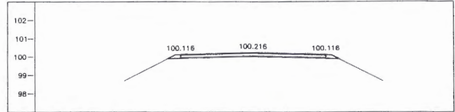
STA. 2+050.000 NGL = 99.905
