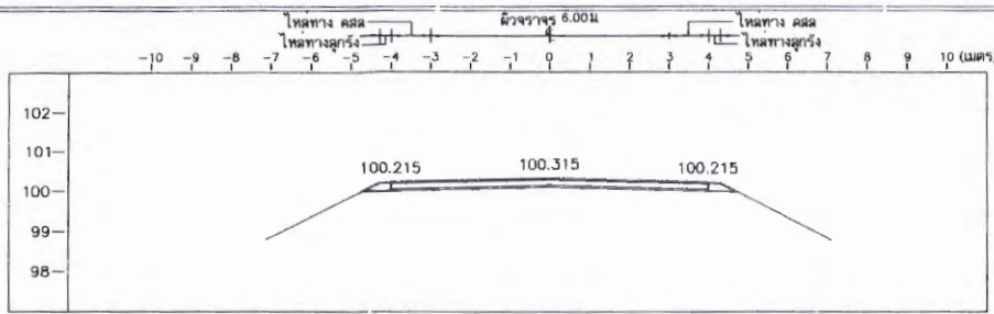
STA. 1+975.000 NGL = 100.014
