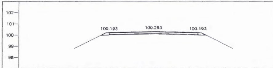
STA. 1+950.000 NGL = 100.036
