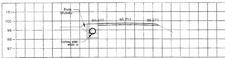
STA. 0+475.000 NGL = 99.442
