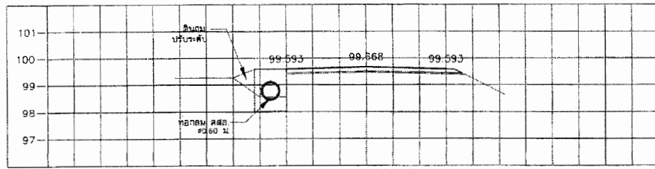
STA. 0+450.000 NGL = 99.345
