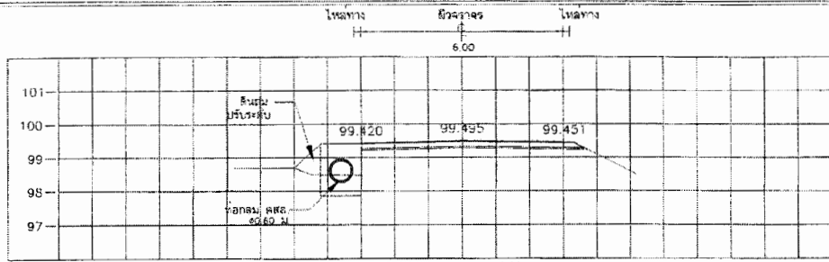
STA. 0+300.000 NGL = 99.100
