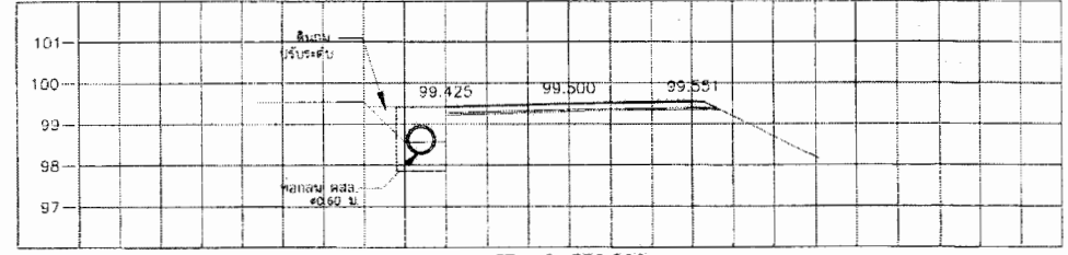
STA. 0+350.000 NGL = 99.132
