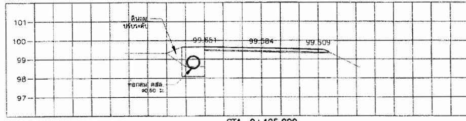
STA. 0+425.000 NGL = 99.270
