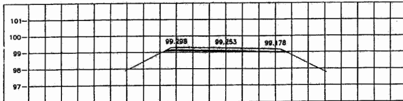
STA. 0+550.000 NGL = 98.932
