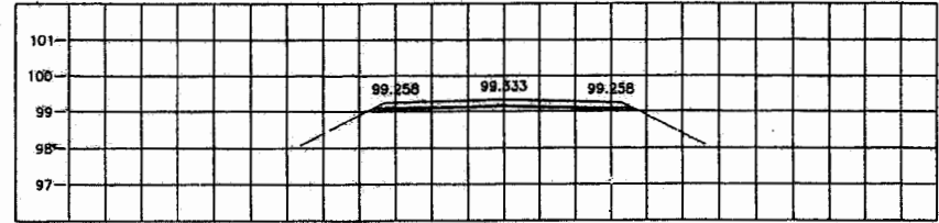
STA. 0+650.000 NGL = 99.083
