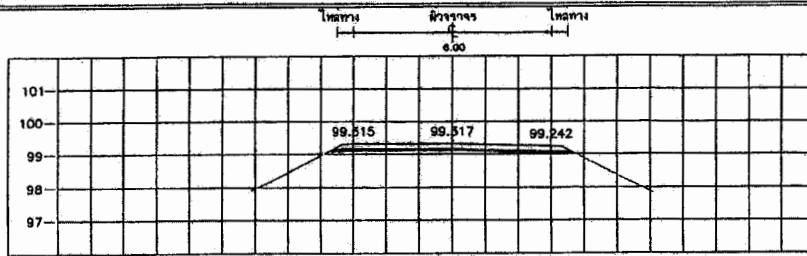
STA. 0+625.000 NGL = 98.954
