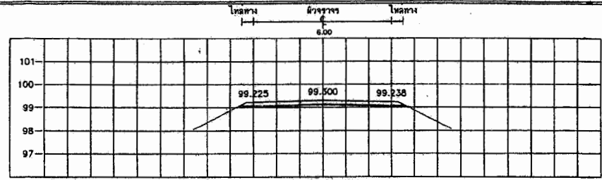
STA. 0+710.000 NGL = 99.089
