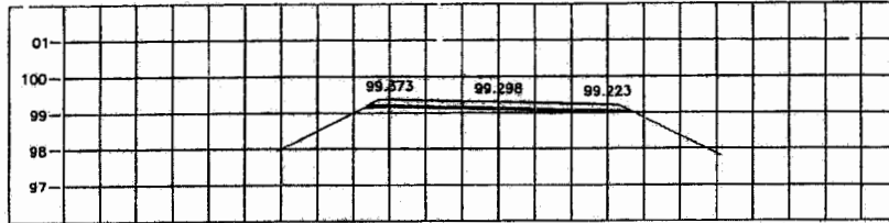
STA. 0+600.000 NGL = 98.858
