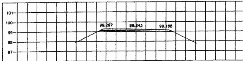
STA. 0+525.000 NGL = 98.727
