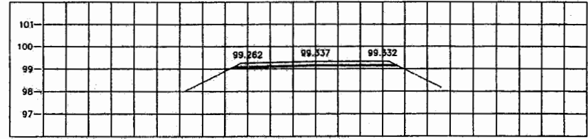
STA. 0+675.000 NGL = 98.920
