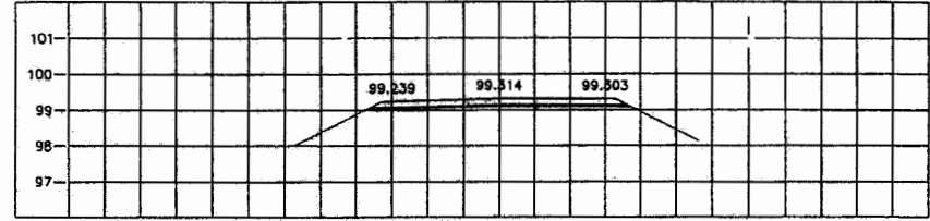
STA. 0+700.000 NGL = 99.039
