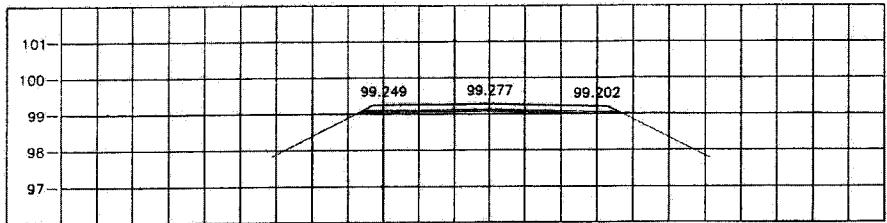
STA. 0+575.000 NGL = 99.022
