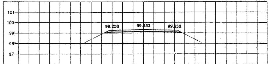
STA. 0+650.000 NGL = 99.083
