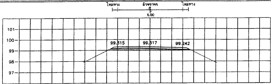
STA. 0+625.000 NGL = 98.954
