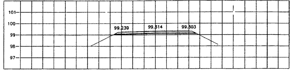
STA. 0+700.000 NGL = 99.039
