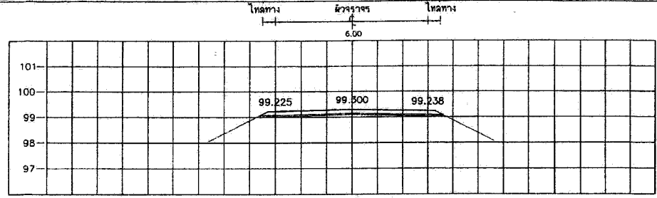
STA. 0+710.000 NGL = 99.089
