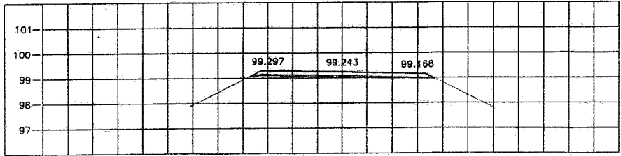
STA. 0+525.000 NGL = 98.727
