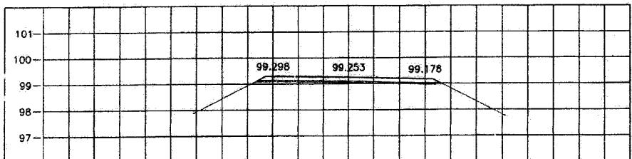
STA. 0+550.000 NGL = 98.932
