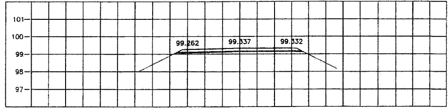
STA. 0+675.000 NGL = 98.920
