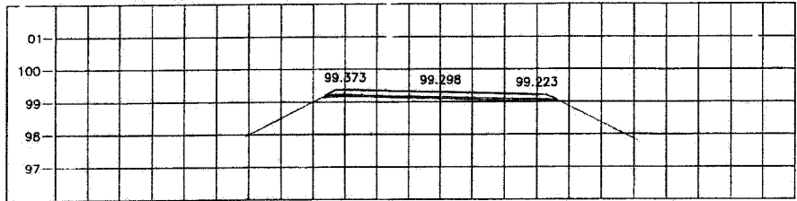
STA. 0+600.000 NGL = 98.958
