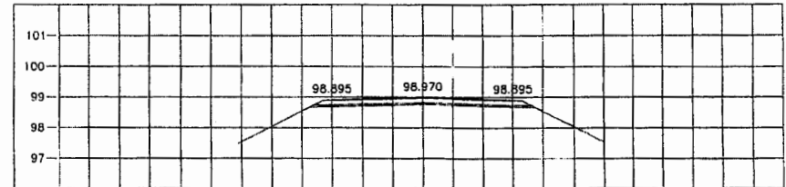
STA. 14+275.000 NGL = 98.638
