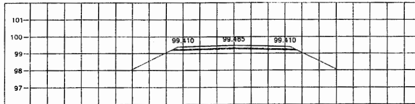
STA. 14+150.000 NGL = 99.186
