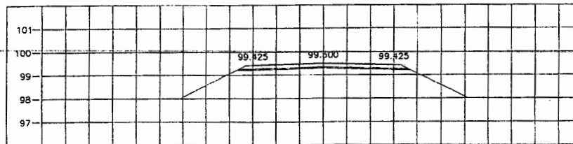
STA. 14+123.000 NGL = 99.296
