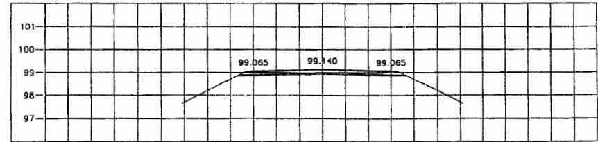
STA. 14+250.000 NGL = 98.726
