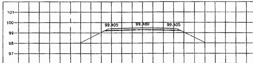
STA. 14+175.000 NGL = 99.279
