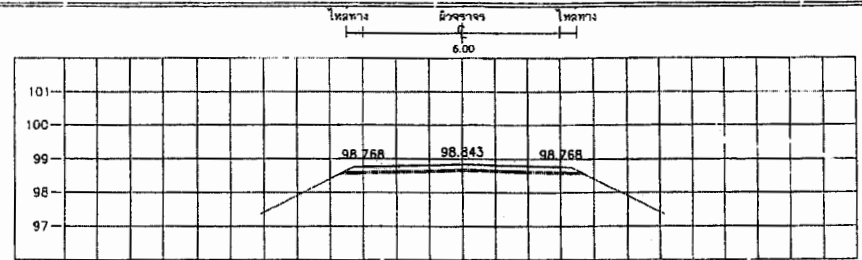
STA. 14+300.000 NGL = 98.503
