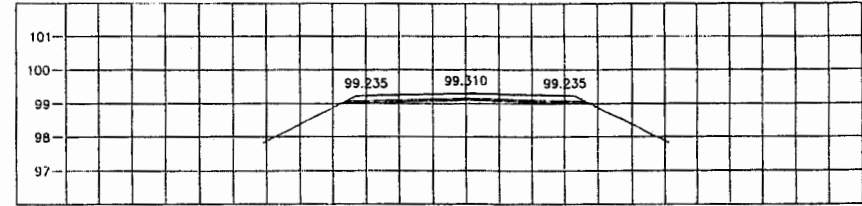
STA. 14+225.000 NGL = 98.936
