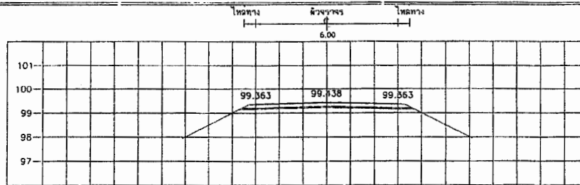
STA. 14+200.000 NGL = 99.187
