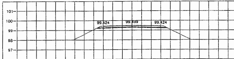
STA. 14+125.000 NGL = 99.246
