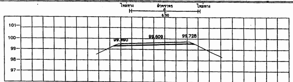
STA. 1+350.000 NGL = 99.336
