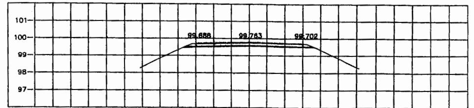
STA. 1+300.000 NGL = 99.413
