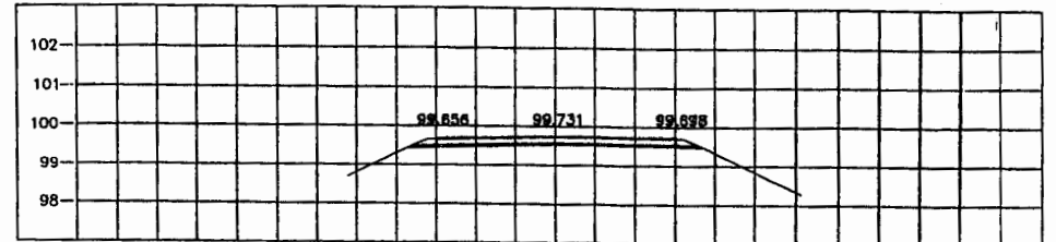
STA. 1+325.000 NGL = 99.509
