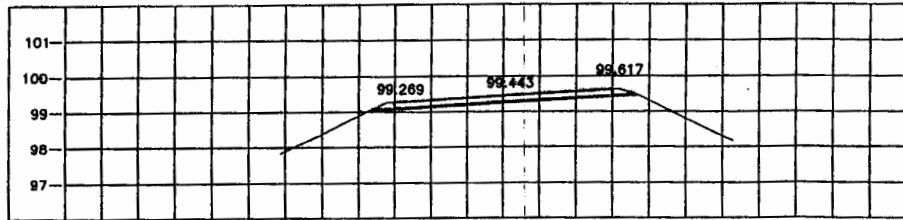
STA. 1+375.000 NGL = 99.144
