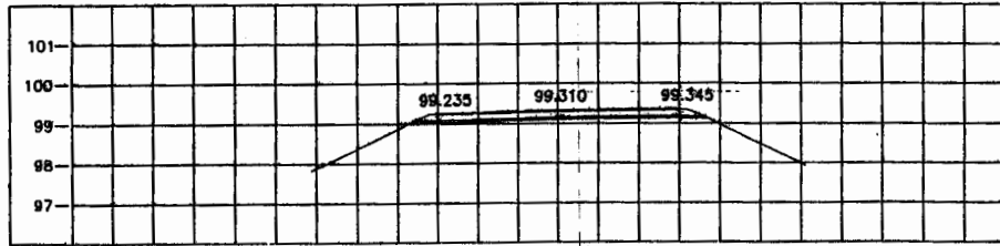
STA. 1+395.000 NGL = 99.130
