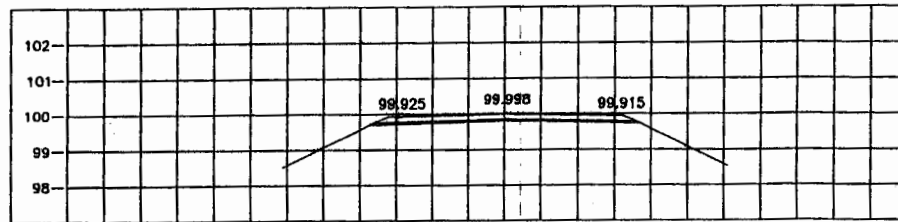
STA. 1+165.000 NGL = 99.998
