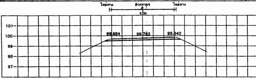
STA. 1+290.000 NGL = 99.457
