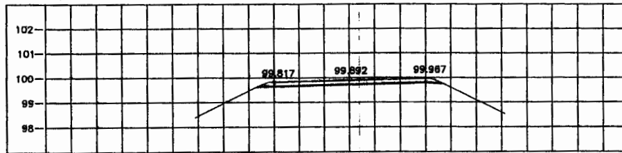
STA. 1+200.000 NGL = 99.576
