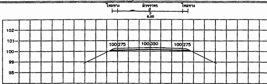
STA. 1+400.000 NGL = 99.958
