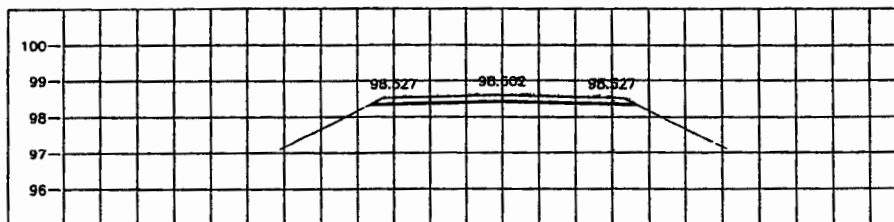
STA. 1+325.000 NGL = 98.324
