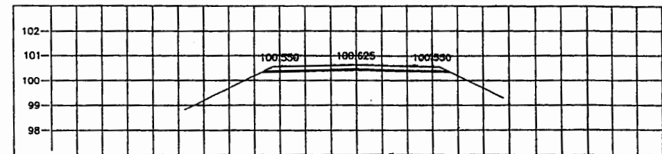
STA. 1+425.000 NGL = 100.324
