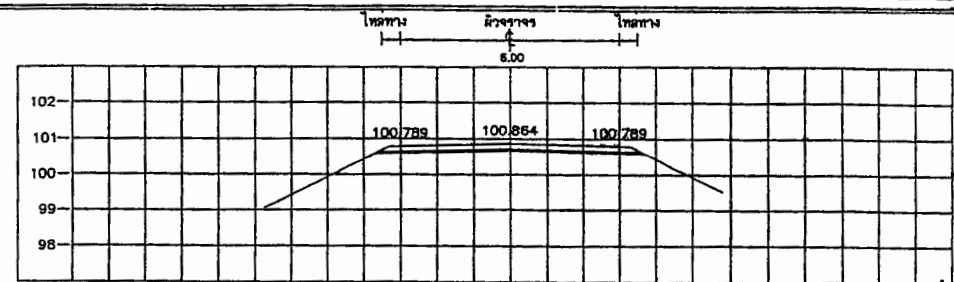
STA. 1+500.000 NGL = 100.452
