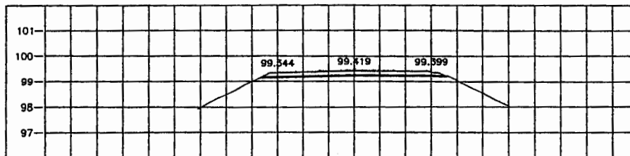
STA. 1+350.000 NGL = 99.123
