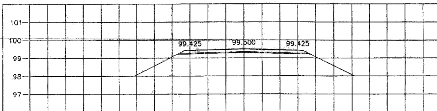
STA. 14+123.000 NGL = 99.296
