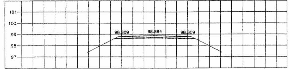
STA. 14+475.000 NGL = 98.528
