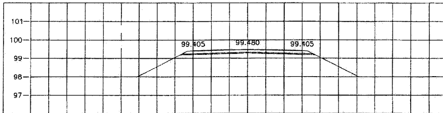
STA. 14+175.000 NGL = 99.279
