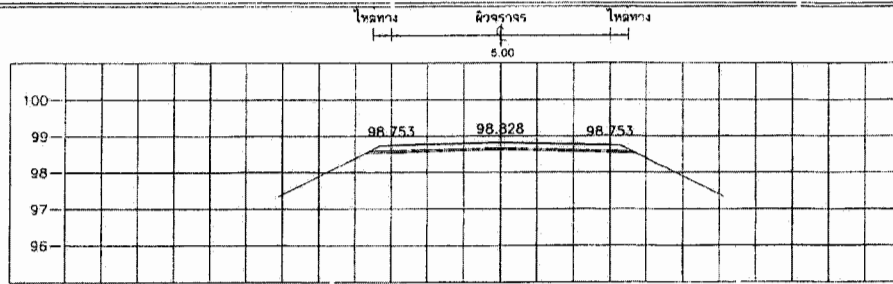
STA. 14+425.000 NGL = 98.458
