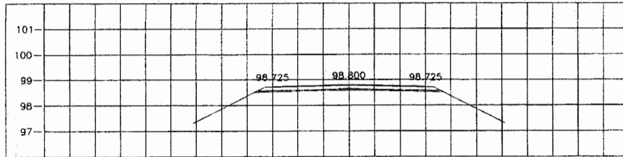
STA. 14+375.000 NGL = 98.593
