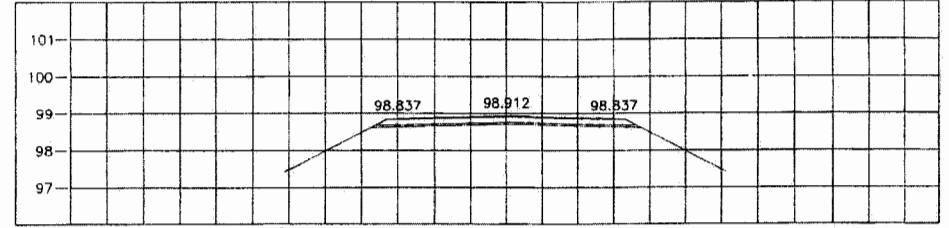
STA. 14+500.000 NGL = 98.534
