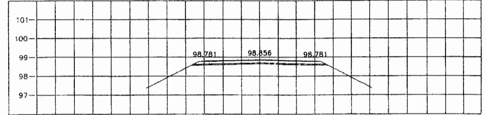
STA. 14+450.000 NGL = 98.525
