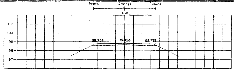
STA. 14+300.000 NGL = 98.503
