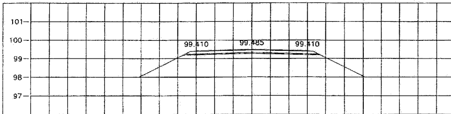
STA. 14+150.000 NGL = 99.186
