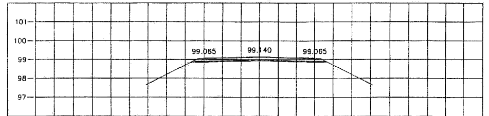
STA. 14+250.000 NGL = 98.726
