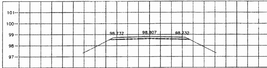
STA. 14+400.000 NGL = 98.503
