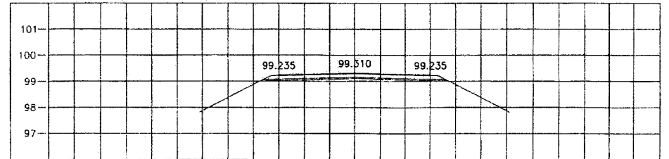
STA. 14+225.000 NGL = 98.936
