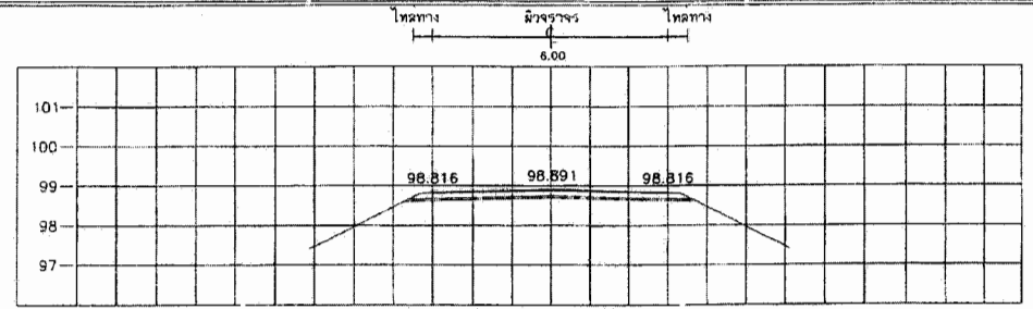
STA. 14+525.000 NGL = 98.638
