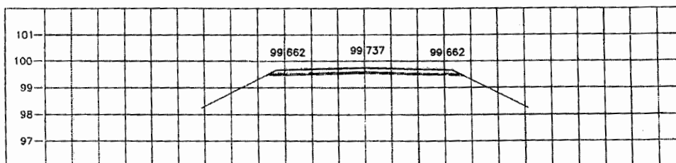
STA. 0+100.000 NGL = 99.301
