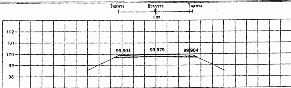
STA. 0+175.000 NGL = 99.580
