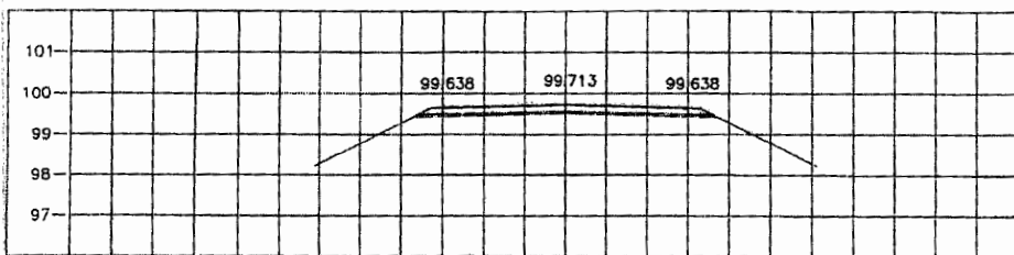
STA. 0+050.000 NGL = 99.270
