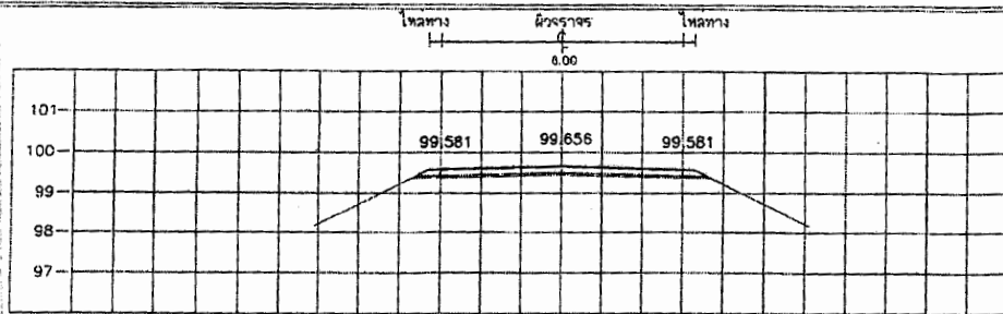
STA. 0+075.000 NGL = 99.226
