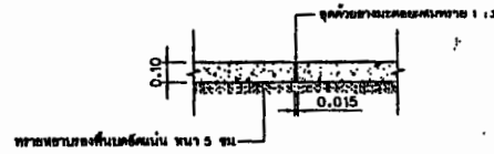
แบบขยายรายละเอียด 2 มาตรฐาน NOT TO SCALE
