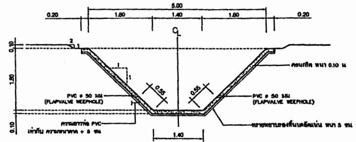
รูปตัด A มาตรฐาน 1 : 50
