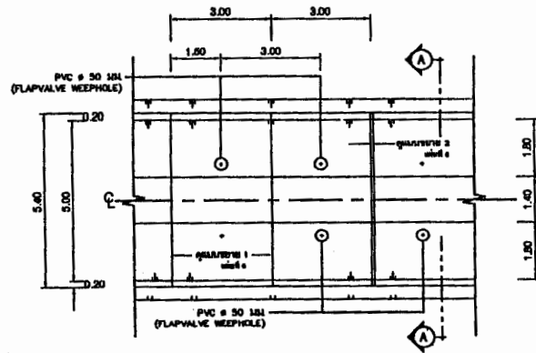
แผนผังโครงตาชั่งคอนกรีต มาตรฐาน 1 : 100
