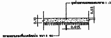
แบบขยายรายละเอียด 1 มาตรฐาน NOT TO SCALE
