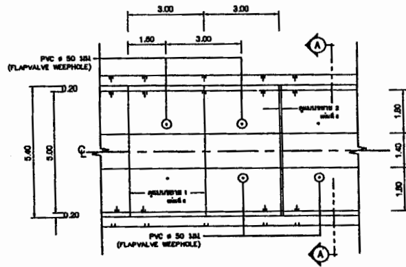
แปลนคลองลาดคอนกรีต มาตราส่วน 1 : 100
