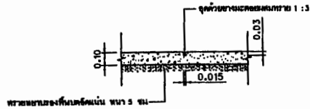
แบบขยายรายละเอียด 1 มาตราส่วน NOT TO SCALE
