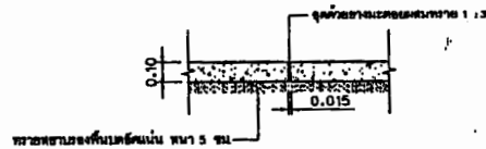
แบบขยายรายละเอียด 2 มาตราส่วน NOT TO SCALE
