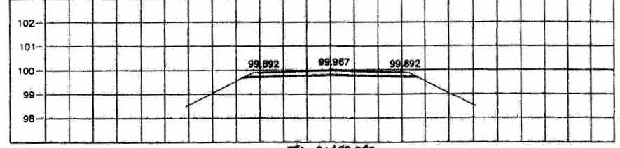
STA. 0+125.000 NGL = 99.537
