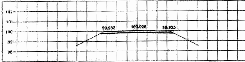
STA. 0+075.000 NGL = 99.739
