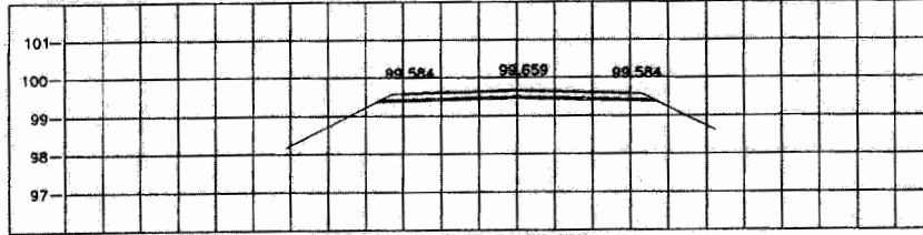
STA. 0+025.000 NGL = 99.401
