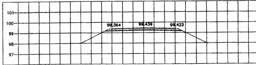
STA. 0+000.000 NGL = 99.439
