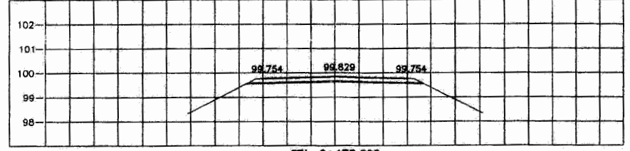
STA. 0+175.000 NGL = 99.500
