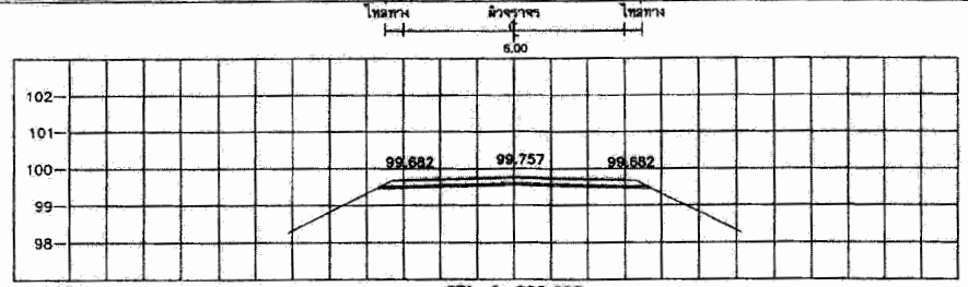
STA. 0+200.000 NGL = 99.527
