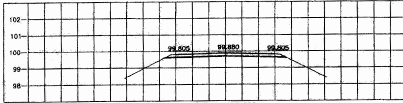
STA. 0+050.000 NGL = 99.599
