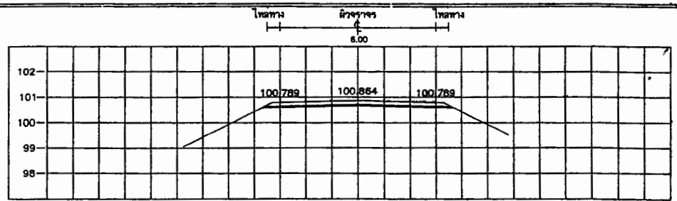
STA. 1+500.000 NGL = 100.452
