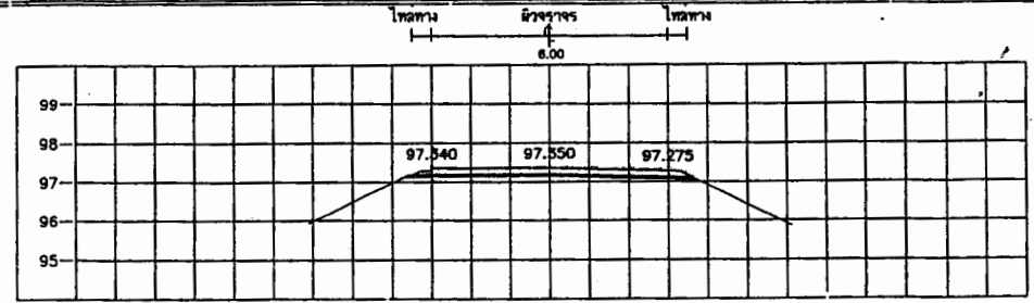
STA. 1+720.000 NGL = 97.059
