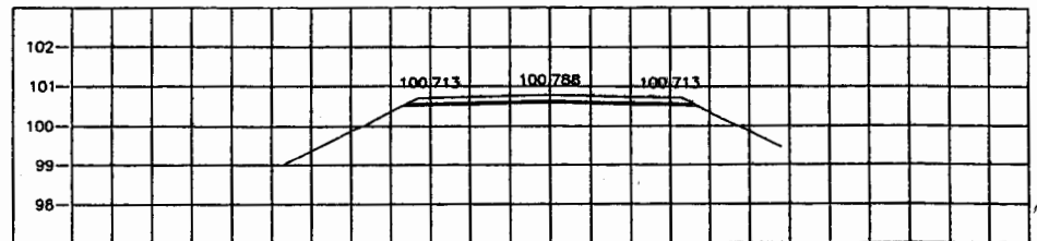
STA. 1+450.000 NGL = 100.404
