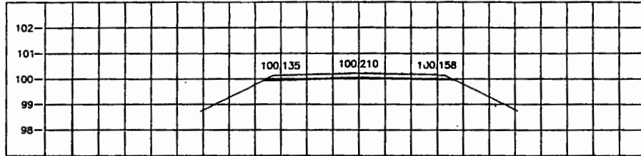
STA. 1+600.000 NGL = 99.706
