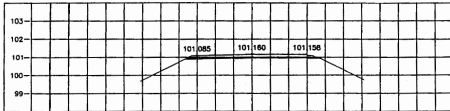
STA. 1+575.000 NGL = 100.804
