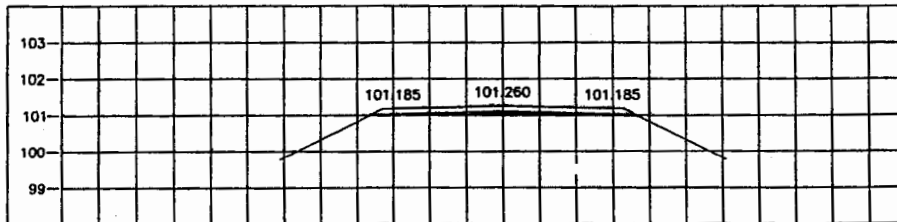
STA. 1+550.000 NGL = 101.022
