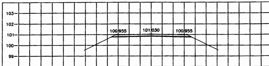
STA. 1+525.000 NGL = 100.509
