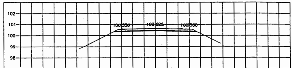
STA. 1+425.000 NGL = 100.324
