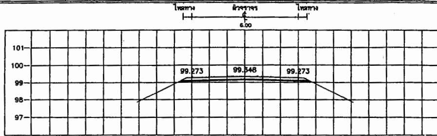
STA. 1+625.000 NGL = 98.927
