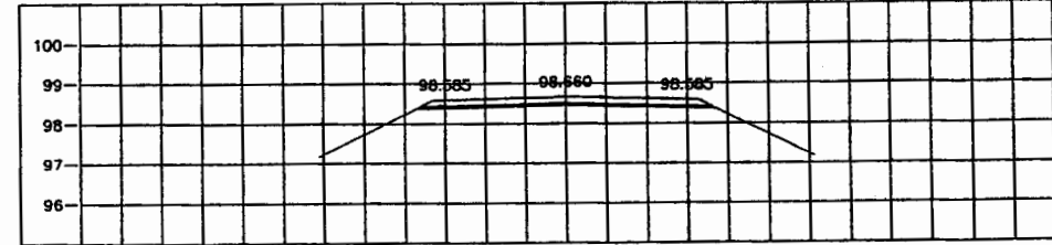
STA. 1+650.000 NGL = 98.349
