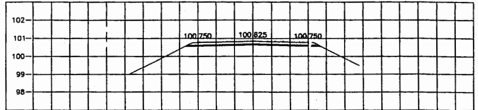
STA. 1+475.000 NGL = 100.249
