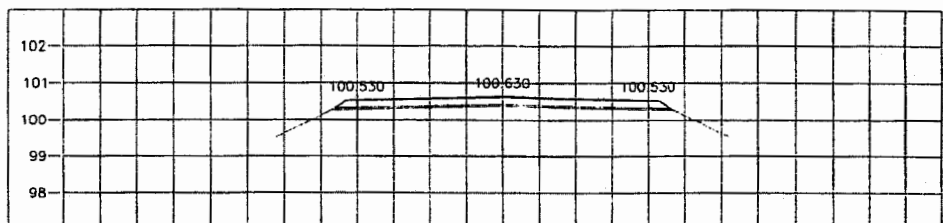
STA. 3+025.000 NGL = 100.475
