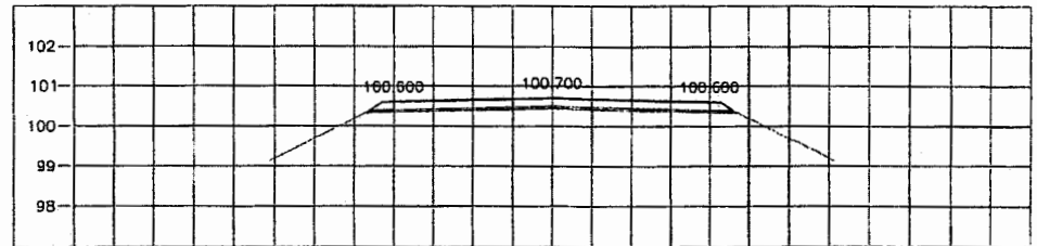
STA. 3+225.000 NGL = 100.483
