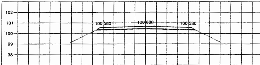
STA. 3+150.000 NGL = 100.482
