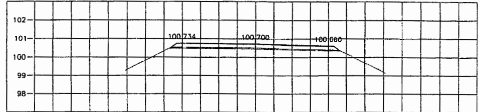
STA. 3+275.000 NGL = 100.412
