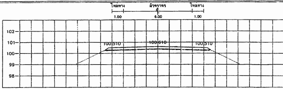
STA. 2+975.000 NGL = 100.359
