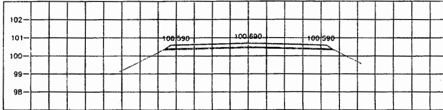
STA. 3+175.000 NGL = 100.492
