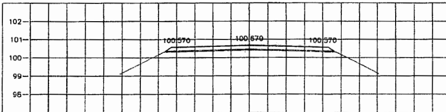
STA. 3+125.000 NGL = 100.468
