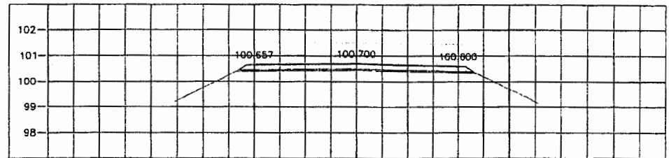
STA. 3+250.000 NGL = 100.470
