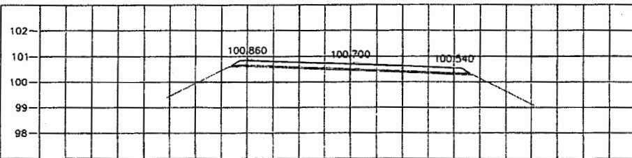
STA. 3+325.000 NGL = 100.352
