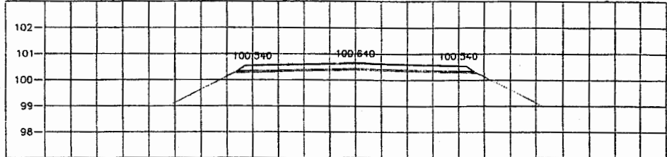
STA. 3+050.000 NGL = 100.492
