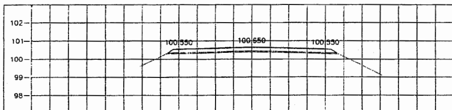
STA. 2+925.000 NGL = 100.368
