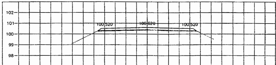
STA. 3+000.000 NGL = 100.429
