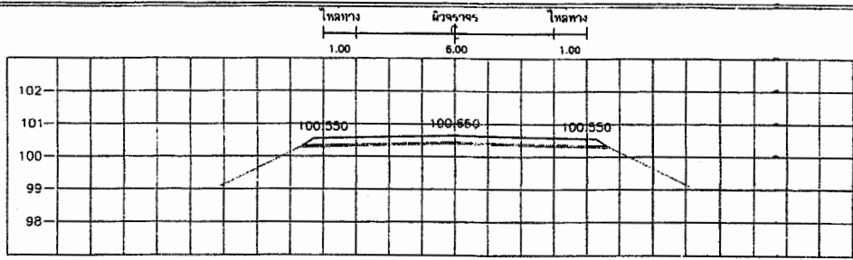
STA. 3+075.000 NGL = 100.474
