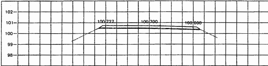
STA. 3+400.000 NGL = 100.476
