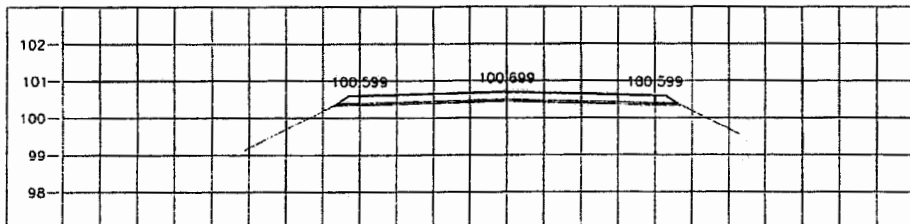
STA. 2+900.000 NGL = 100.407
