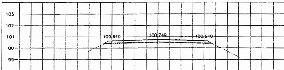
STA. 2+875.000 NGL = 100.505
