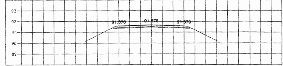
STA. 0+575.000 NGL = 91.418
