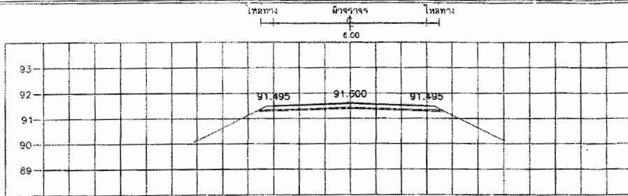
STA. 0+550.000 NGL = 91.280
