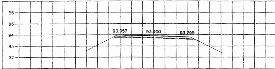
STA. 0+300.000 NGL = 93.702
