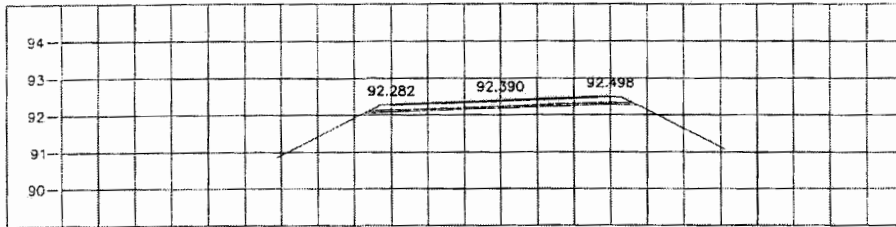
STA. 0+750.000 NGL = 92.326
