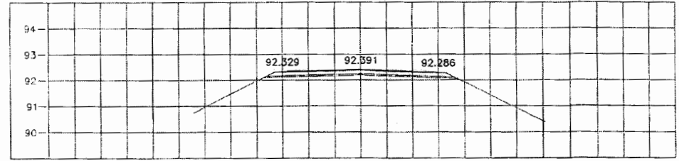
STA. 0+375.000 NGL = 92.174
