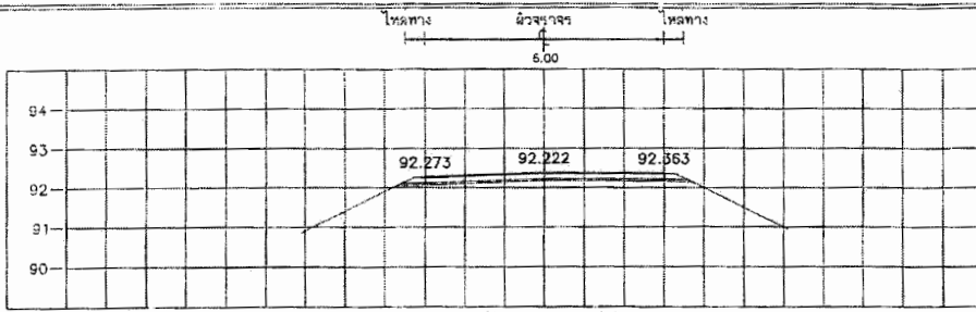
STA. 0+771.000 NGL = 92.172
