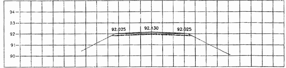
STA. 0+400.000 NGL = 91.849
