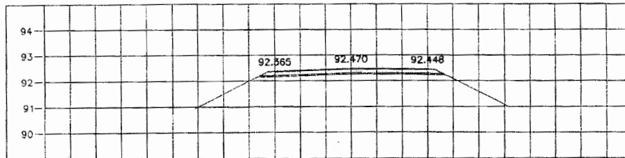
STA. 0+700.000 NGL = 92.106
