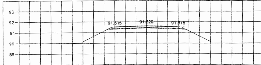
STA. 0+475.000 NGL = 91.379
