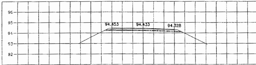
STA. 0+275.000 NGL = 94.207
