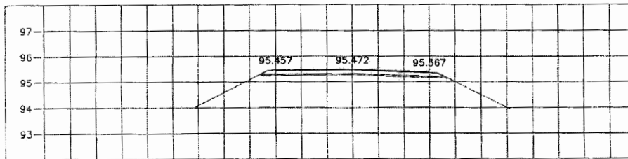
STA. 0+225.000 NGL = 95.363
