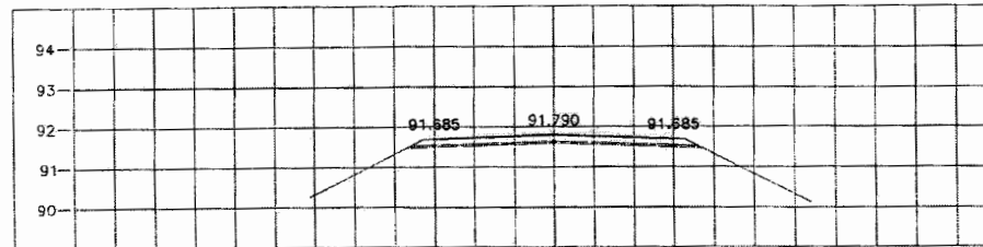
STA. 0+450.000 NGL = 91.547
