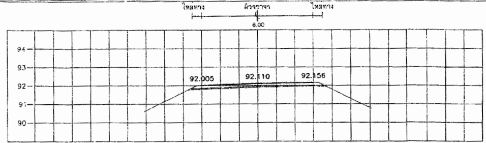
STA. 0+650.000 NGL = 91.790
