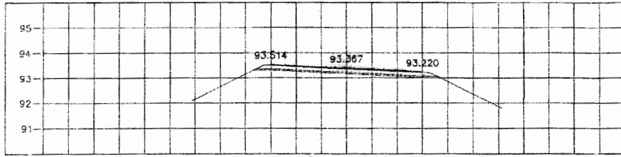
STA. 0+325.000 NGL = 93.183
