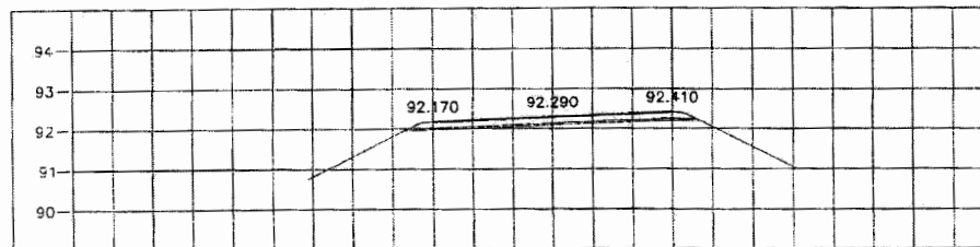
STA. 0+675.000 NGL = 91.934
