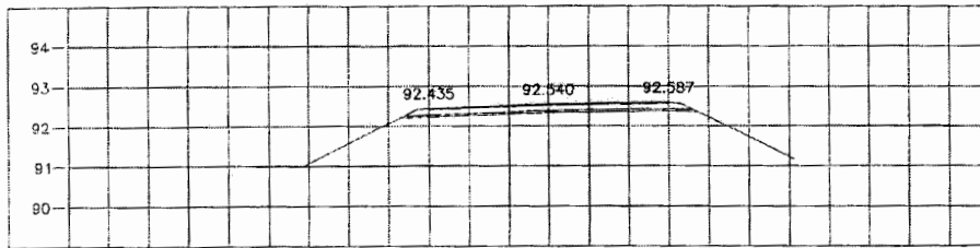
STA. 0+725.000 NGL = 92.343
