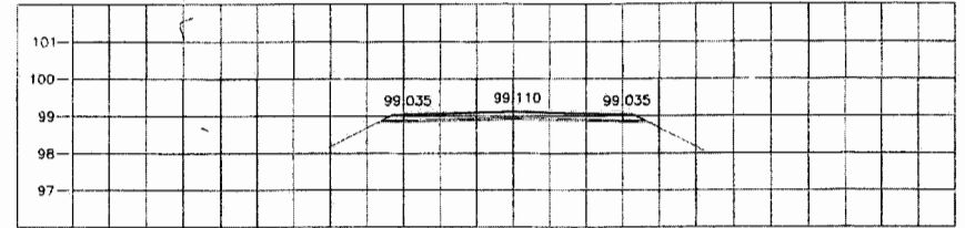
STA. 0+830.000 NGL = 98.895
