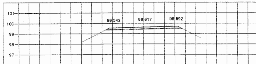
STA. 0+675.000 NGL = 99.246
