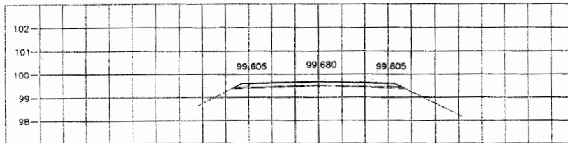
STA. 0+450.000 NGL = 99.538
