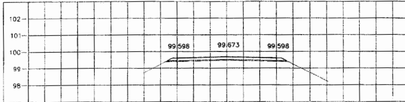
STA. 0+475.000 NGL = 99.505
