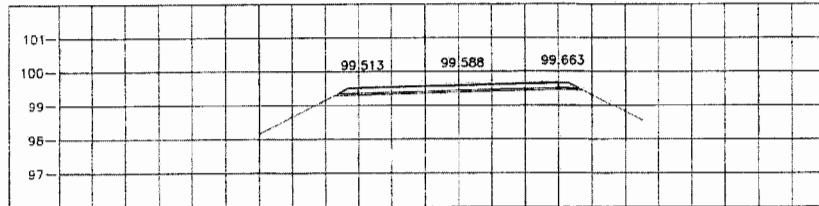
STA. 0+700.000 NGL = 99.264
