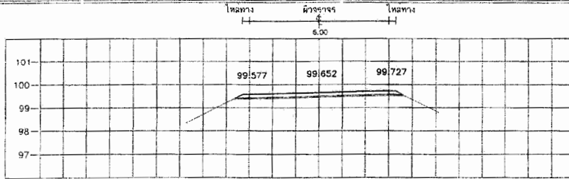
STA. 0+550.000 NGL = 99.356
