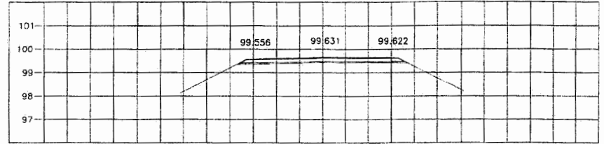
STA. 0+625.000 NGL = 99.127
