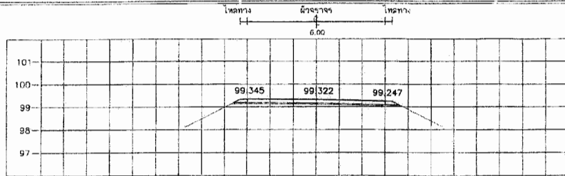
STA. 0+775.000 NGL = 98.907
