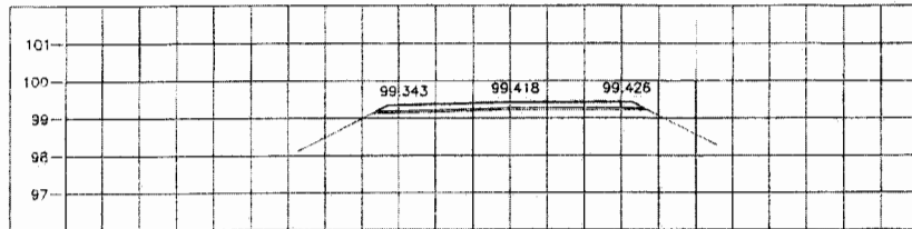
STA. 0+750.000 NGL = 99.027
