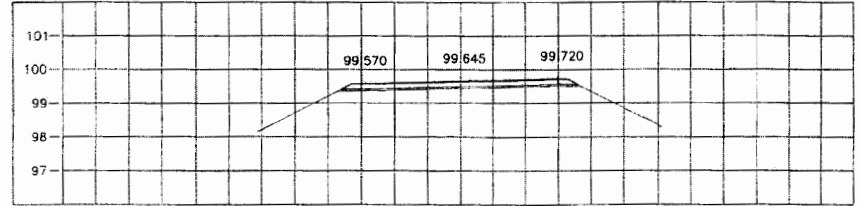
STA. 0+575.000 NGL = 99.227
