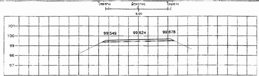
STA. 0+650.000 NGL = 99.214
