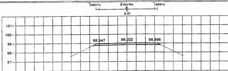
STA. 1+525.000 NGL = 98.788
