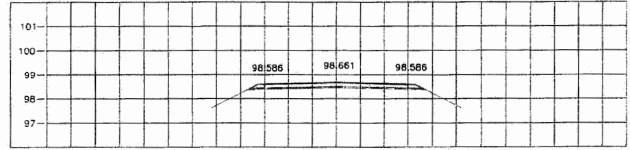
STA. 1+575.000 NGL = 98.658
