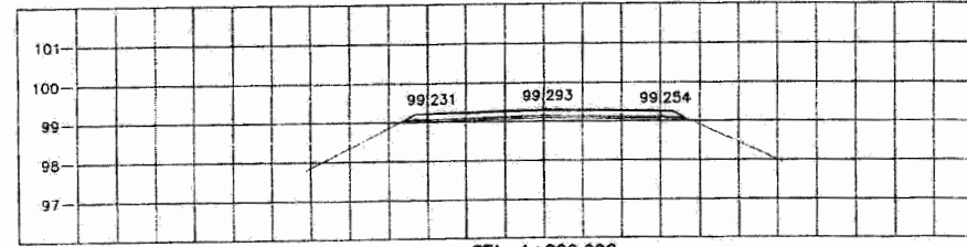
STA. 1+200.000 NGL = 99.293
