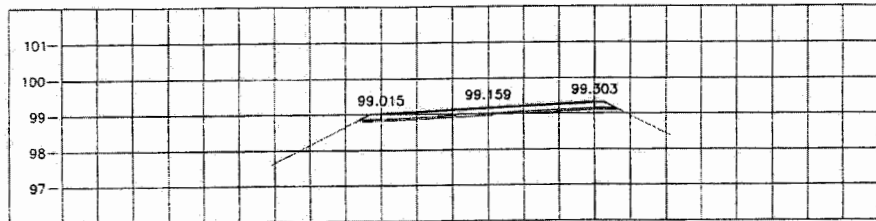
STA. 1+500.000 NGL = 98.842
