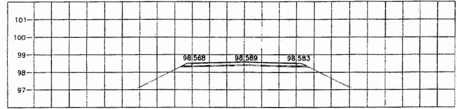
STA. 1+585.000 NGL = 98.589
