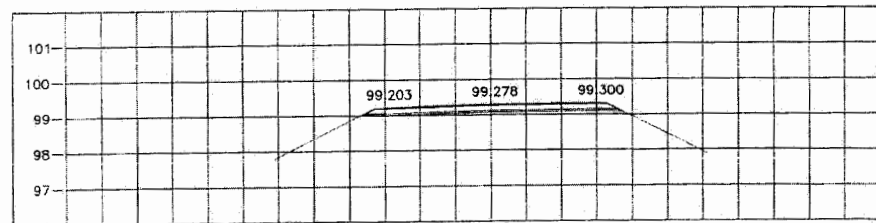
STA. 1+250.000 NGL = 99.007
