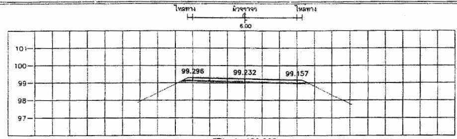
STA. 1+400.000 NGL = 98.838
