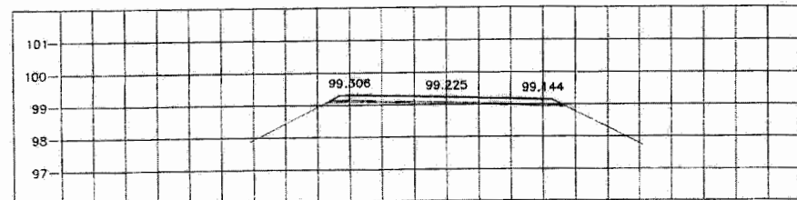
STA. 1+425.000 NGL = 98.887
