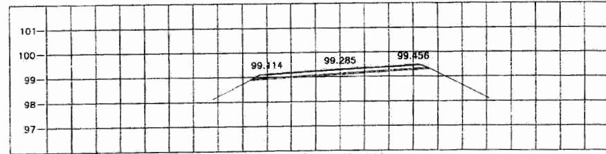
STA. 1+225.000 NGL = 99.127
