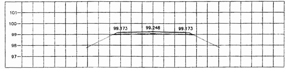
STA. 1+350.000 NGL = 98.869
