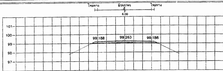
STA. 1+300.000 NGL = 98.861
