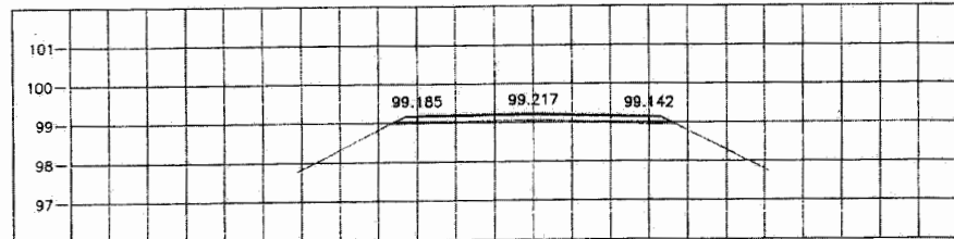
STA. 1+450.000 NGL = 98.857
