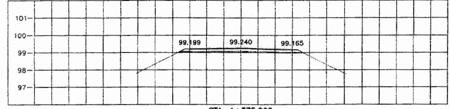
STA. 1+375.000 NGL = 98.831
