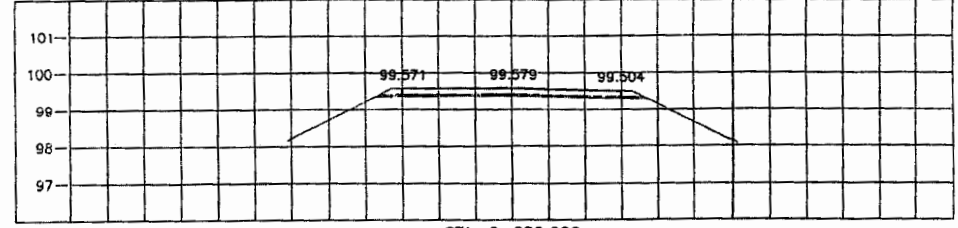
STA. 0+650.000 NGL = 99.292
