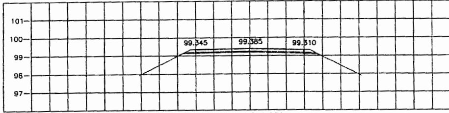
STA. 0+800.000 NGL = 99.102
