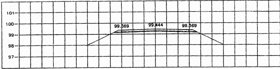
STA. 0+825.000 NGL = 99.202
