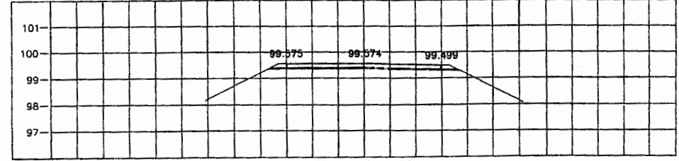
STA. 0+625.000 NGL = 99.339
