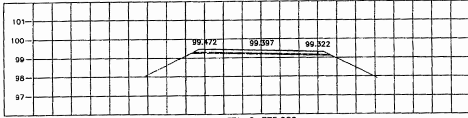
STA. 0+775.000 NGL = 99.088
