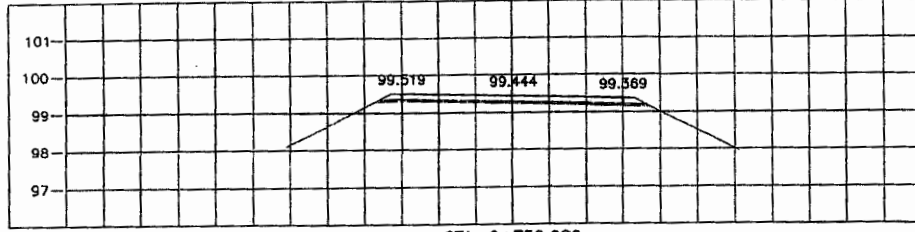
STA. 0+750.000 NGL = 99.152
