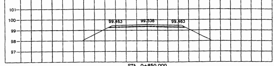
STA. 0+850.000 NGL = 99.327
