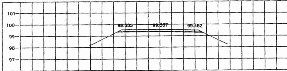
STA. 0+550.000 NGL = 99.374
