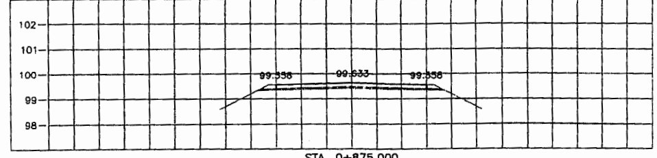
STA. 0+875.000 NGL = 99.620
