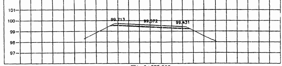
STA. 0+675.000 NGL = 99.444
