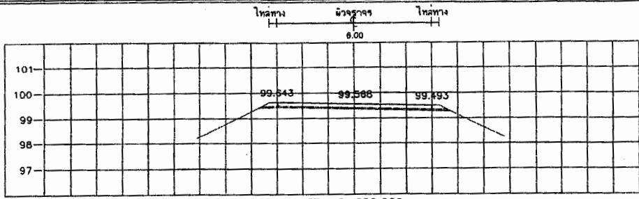
STA. 0+600.000 NGL = 99.249
