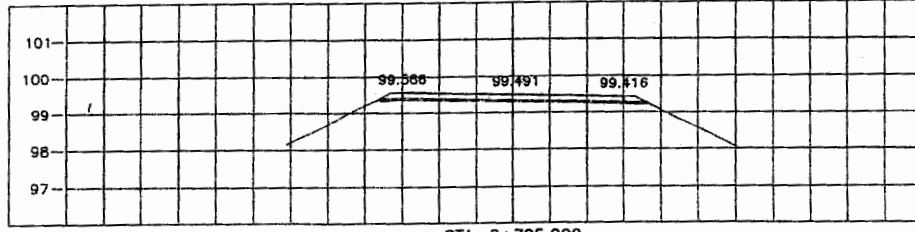
STA. 0+725.000 NGL = 99.156
