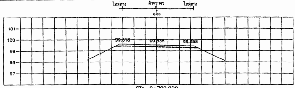
STA. 0+700.000 NGL = 99.317
