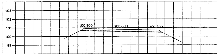
STA. 3+850.000 NGL = 100.610
