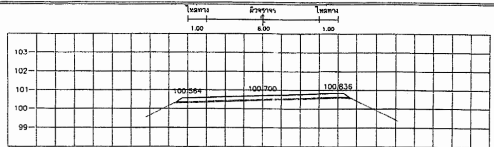
STA 3+525.000 NGL = 100.540
