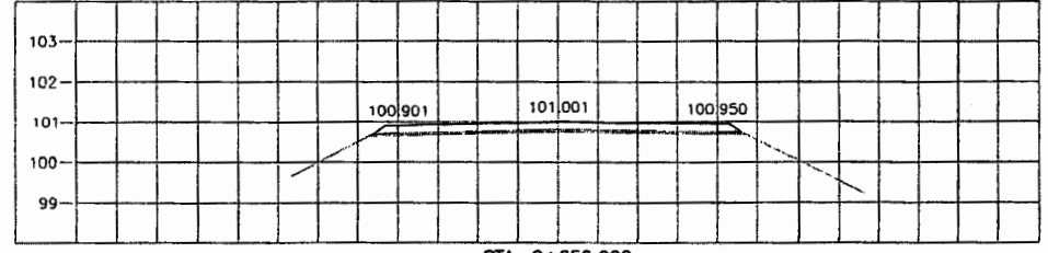
STA. 2+650.000 NGL = 100.847
