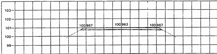
STA. 2+750.000 NCL = 100.963
