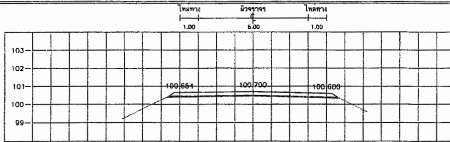
STA 3+425.000 NGL = 100.530
