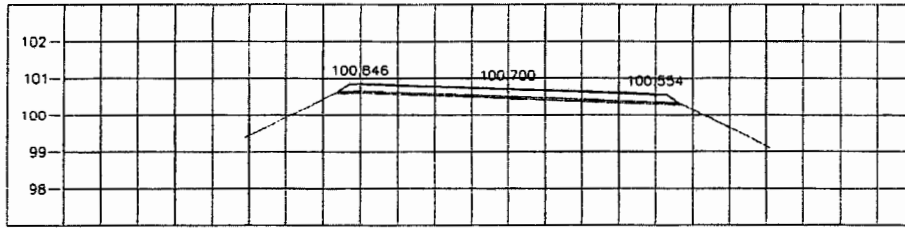
STA 3+375.000 NGL = 100.440
