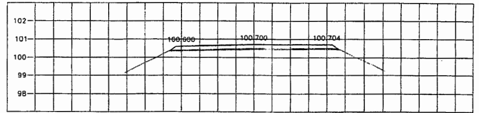
STA 3+475.000 NGL = 100.490
