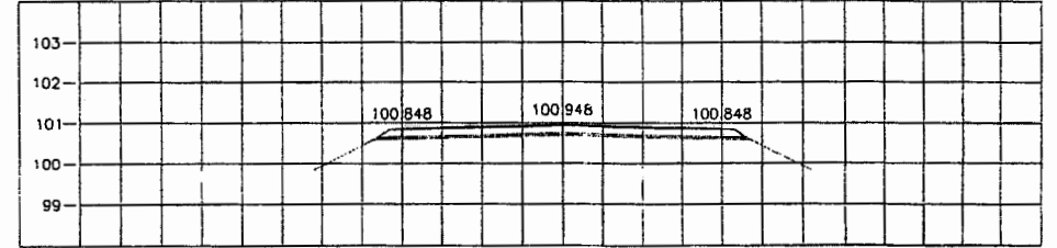
STA. 2+775.000 NCL = 100.838
