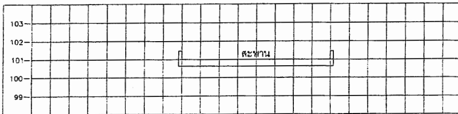
STA. 2+704.000 NCL = 101.002
