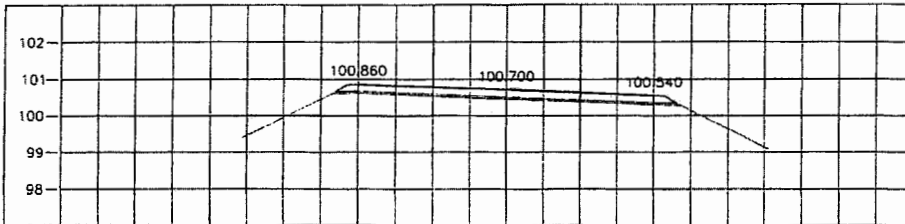
STA 3+325.000 NGL = 100.352
