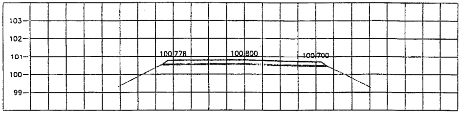
STA. 3+925.000 NGL = 100.580
