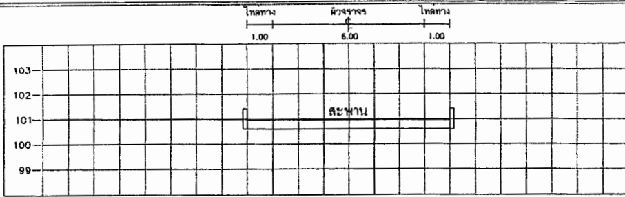
STA. 2+766.000 NCL = 100.966
