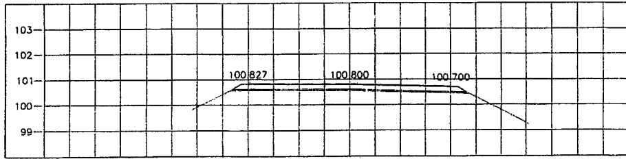
STA. 3+800.000 NGL = 100.546
