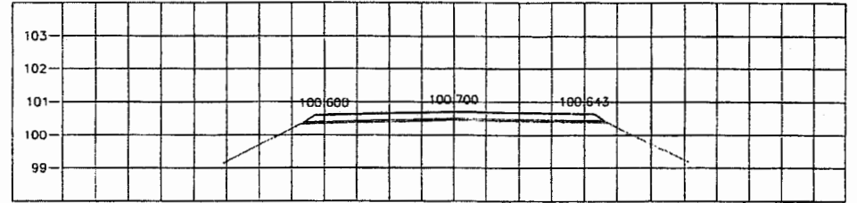
STA 3+450.000 NGL = 100.510
