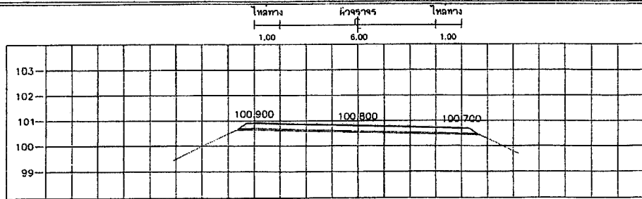
STA. 3+875.000 NGL = 100.604
