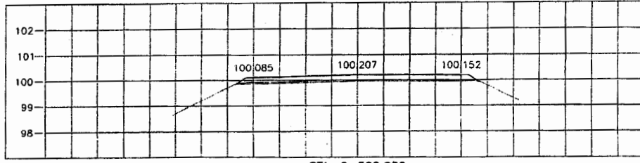
STA. 2+500.000 NGL = 100.207
