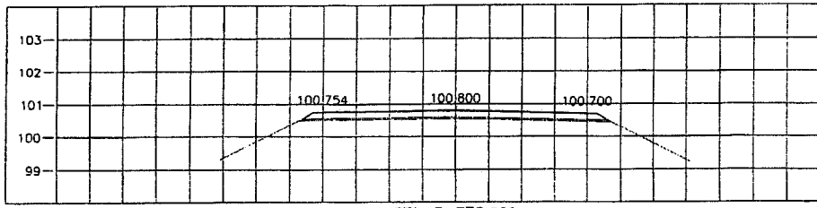
STA. 3+775.000 NGL = 100.564
