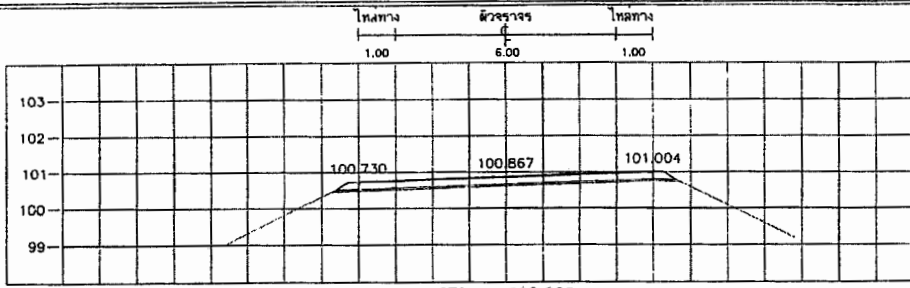
STA. 2+600.000 NGL = 100.582
