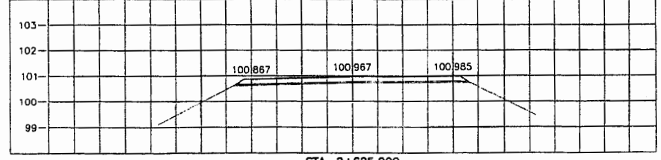
STA. 2+625.000 NGL = 100.737
