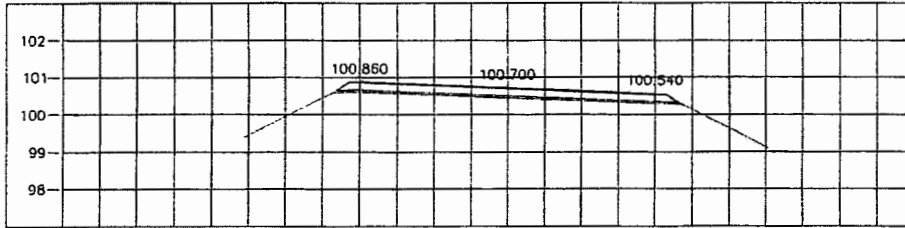
STA 3+350.000 NGL = 100.430
