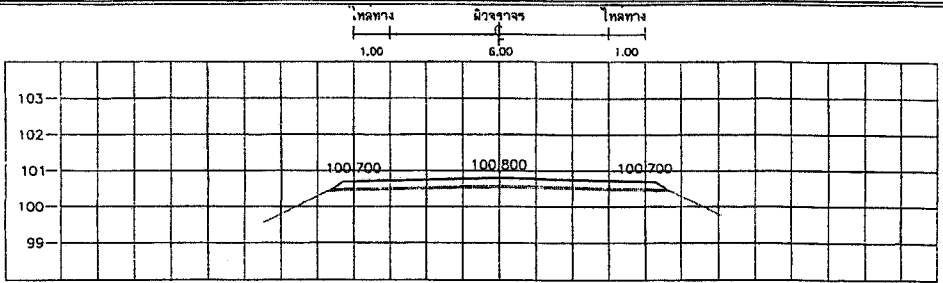
STA. 3+975.000 NGL = 100.604
