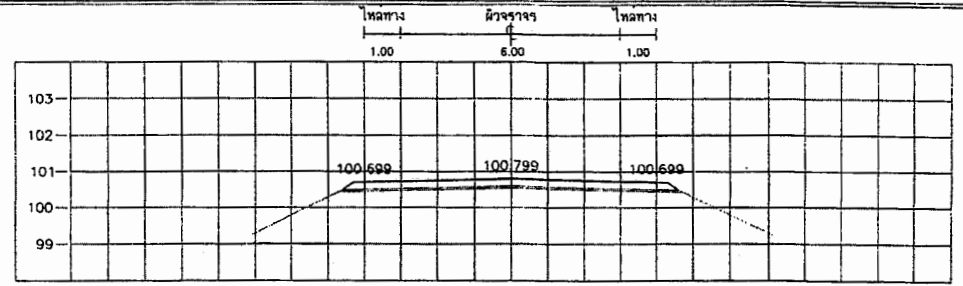
STA. 2+850.000 NCL = 100.588
