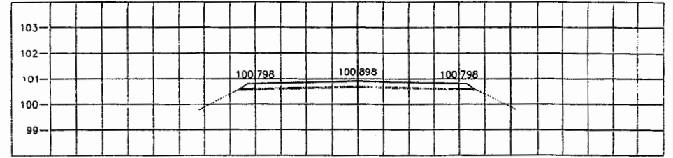
STA. 2+800.000 NCL = 100.723
