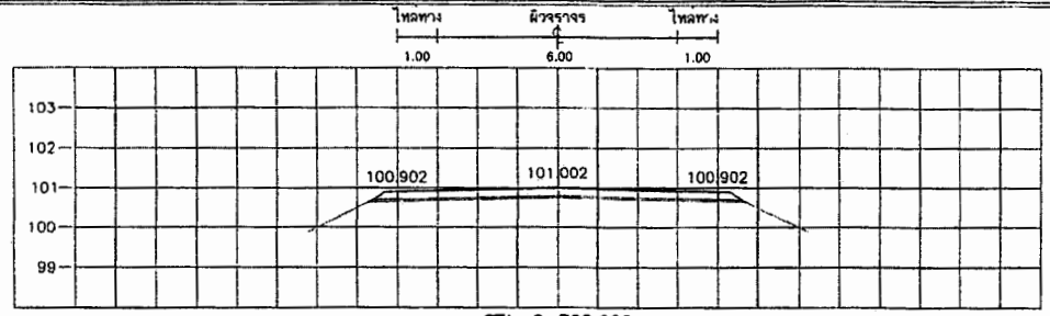
STA. 2+700.000 NGL = 100.891
