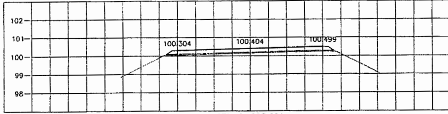
STA. 2+525.000 NGL = 100.253
