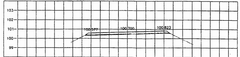
STA 3+500.000 NGL = 100.542
