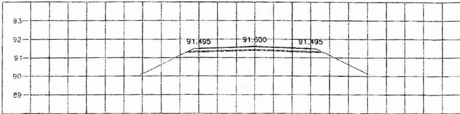
STA. 0+550.000 NGL = 91.280
