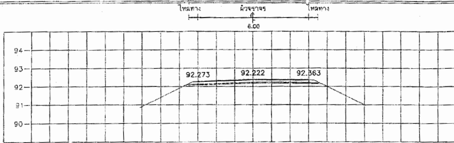
STA. 0+771.000 NGL = 92.172
