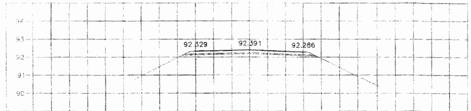
STA. 0+375.000 NGL = 92.174
