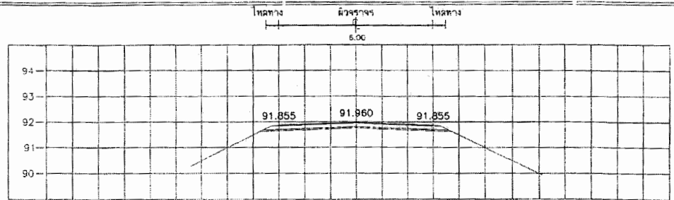
STA. 0+425.000 NGL = 91.684
