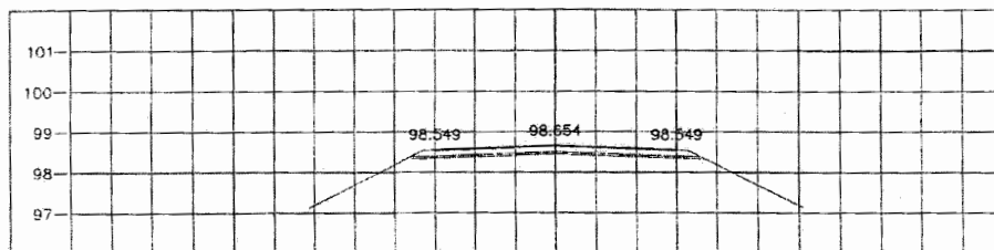
STA. 0+021.000 NGL = 98.654
