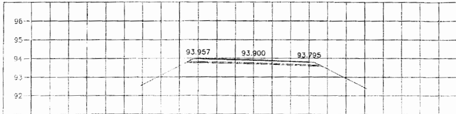
STA. 0+300.000 NGL = 93.702
