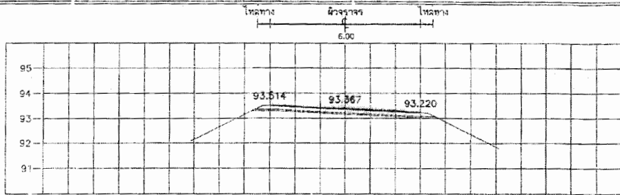
STA. 0+325.000 NGL = 93.163
