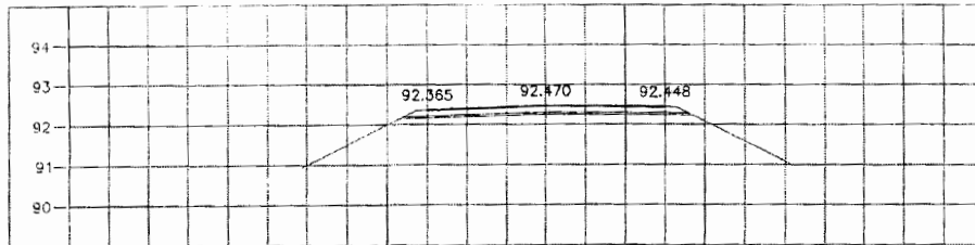
STA. 0+700.000 NGL = 92.106
