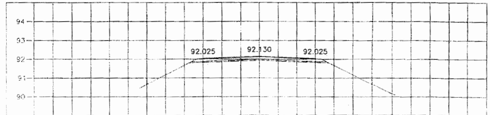
STA. 0+400.000 NGL = 91.849
