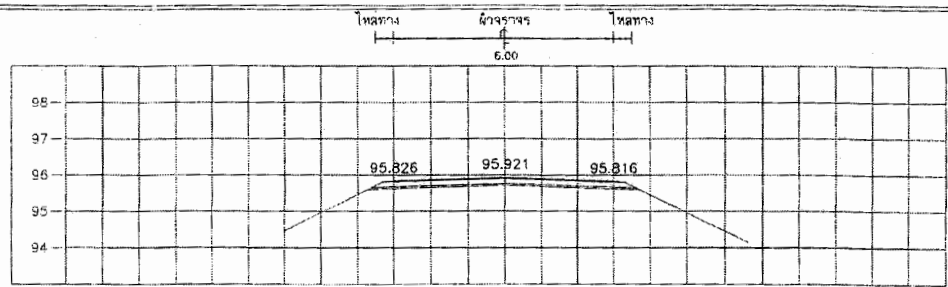
STA. 0+200.000 NGL = 95.773
