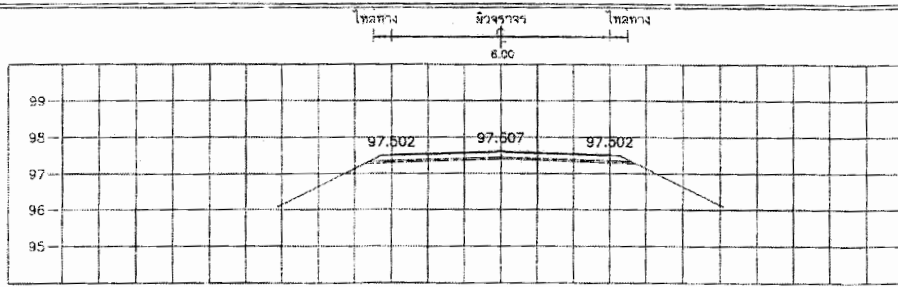
STA. 0+100.000 NGL = 97.390
