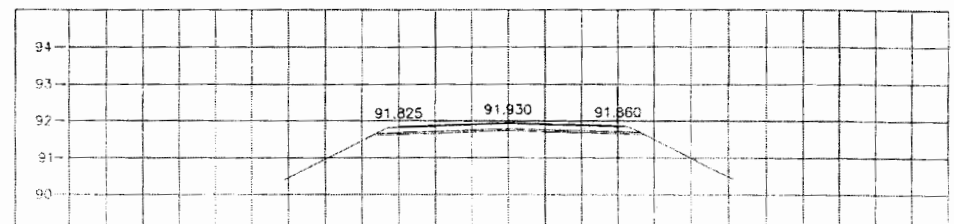
STA. 0+625.000 NGL = 91.609
