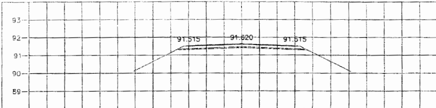
STA. 0+475.000 NGL = 91.379
