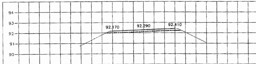
STA. 0+675.000 NGL = 91.934
