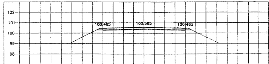
STA. 3+925.000 NGL = 100.292
