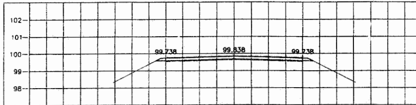
STA. 3+175.000 NGL = 99.622
