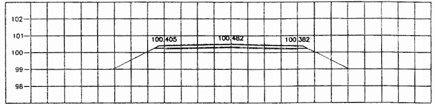
STA. 3+475.000 NGL = 100.178
