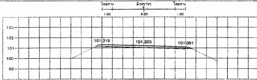
STA. 4+325.000 NGL = 100.910
