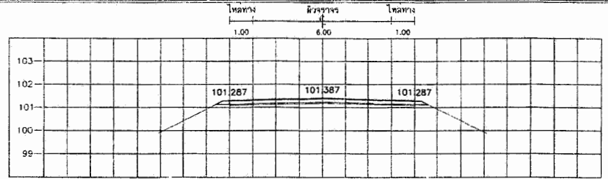
STA. 4+425.000 NGL = 101.128
