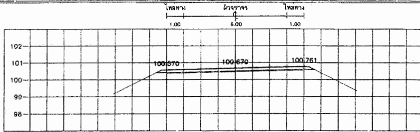
STA. 3+650.000 NGL = 100.414
