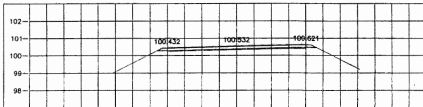
STA. 3+575.000 NGL = 100.259
