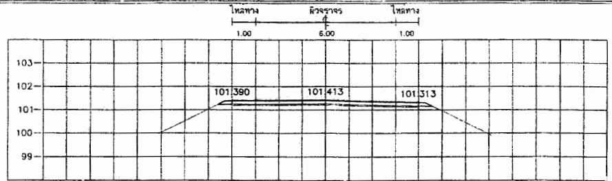
STA. 4+650.000 NGL = 101.117
