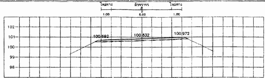
STA. 4+200.000 NGL = 100.495
