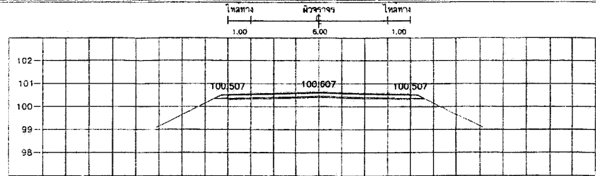
STA. 3+975.000 NGL = 100.283
