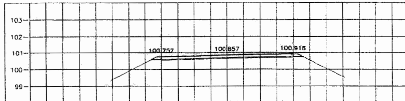
STA. 4+225.000 NGL = 100.505
