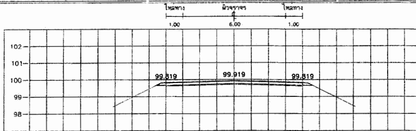
STA. 3+200.000 NGL = 99.673
