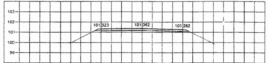
STA. 4+400.000 NGL = 101.127
