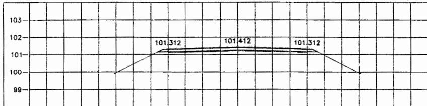
STA. 4+475.000 NGL = 101.153
