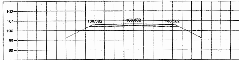
STA. 4+050.000 NGL = 100.347
