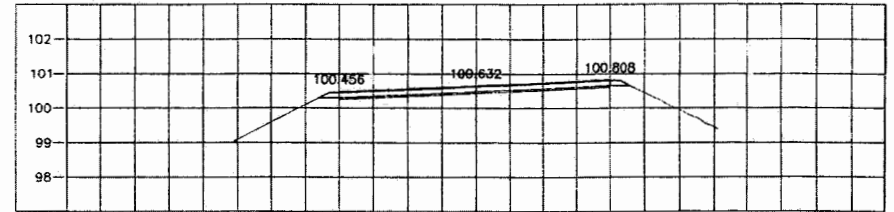
STA. 3+725.000 NGL = 100.261
