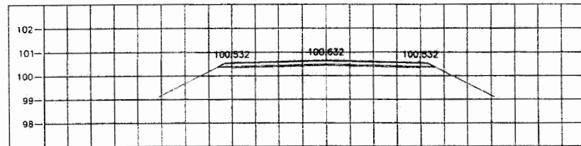
STA. 4+000.000 NGL = 100.341
