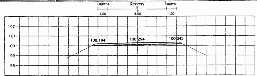
STA. 3+300.000 NGL = 100.043
