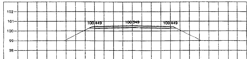
STA. 3+900.000 NGL = 100.257
