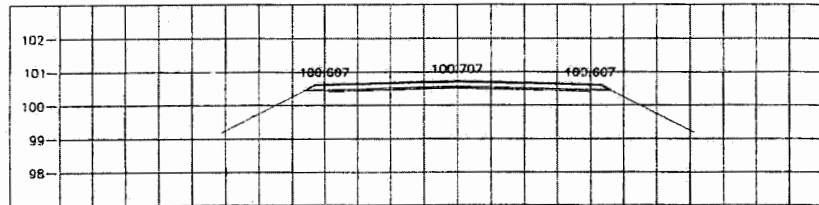
STA. 4+075.000 NGL = 100.393
