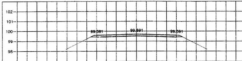
STA. 3+125.000 NGL = 99.543
