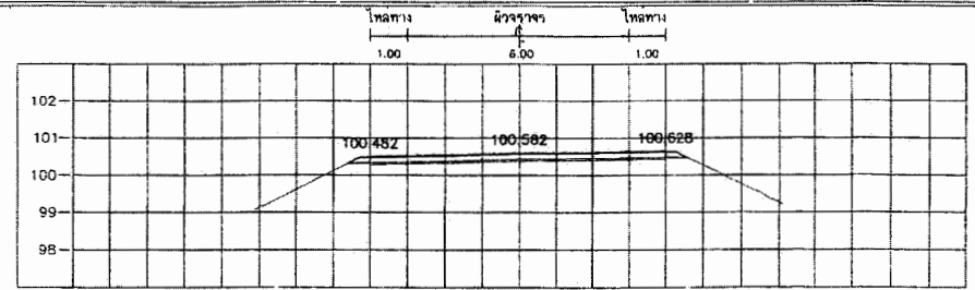
STA. 3+750.000 NGL = 100.160
