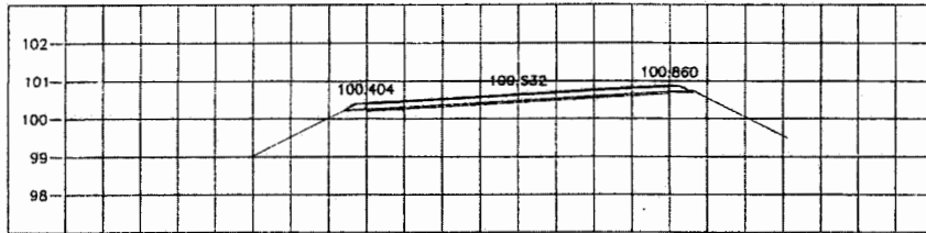
STA. 3+825.000 NGL = 100.369
