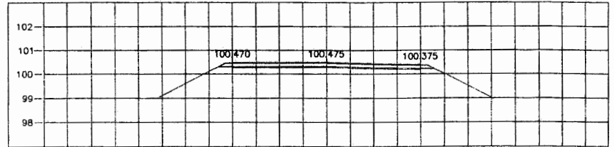
STA. 3+450.000 NGL = 100.163
