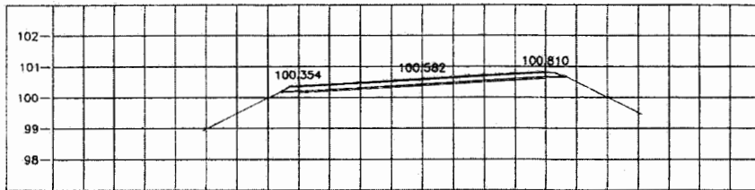
STA. 3+600.000 NGL = 100.288
