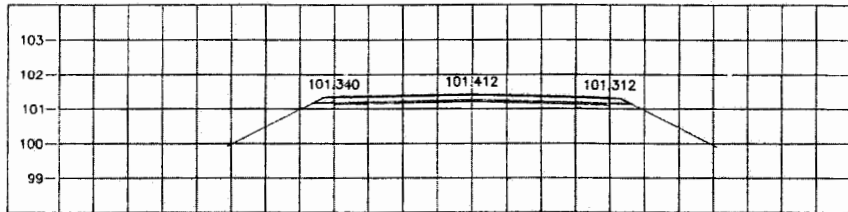
STA. 4+525.000 NGL = 101.118
