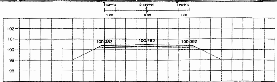
STA. 3+525.000 NGL = 100.171
