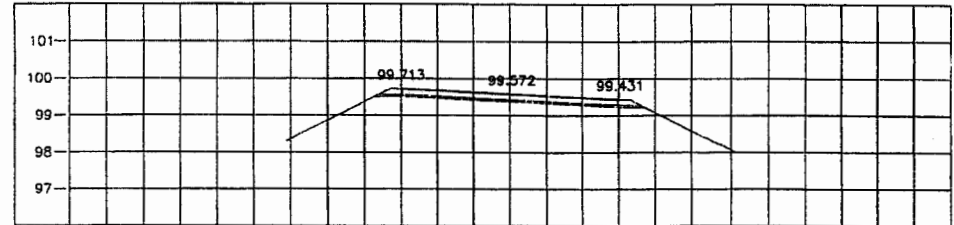
STA. 0+675.000 NGL = 99.444
