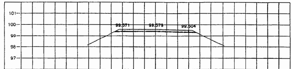
STA. 0+650.000 NGL = 99.292
