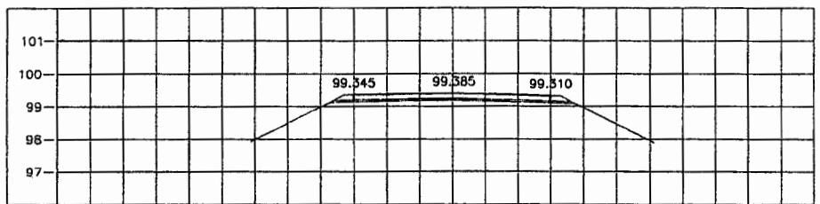
STA. 0+800.000 NGL = 99.102
