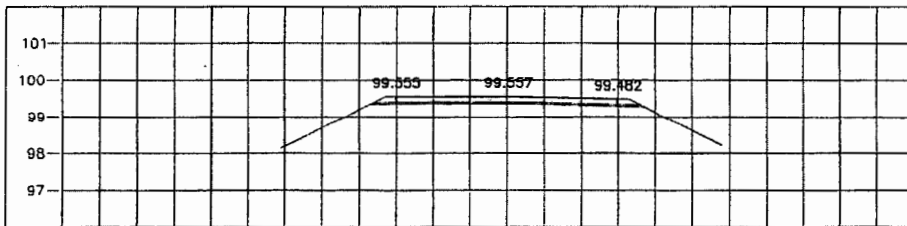
STA. 0+550.000 NGL = 99.374
