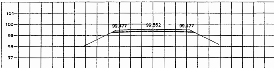
STA. 0+525.000 NGL = 99.310
