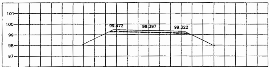
STA. 0+775.000 NGL = 99.088
