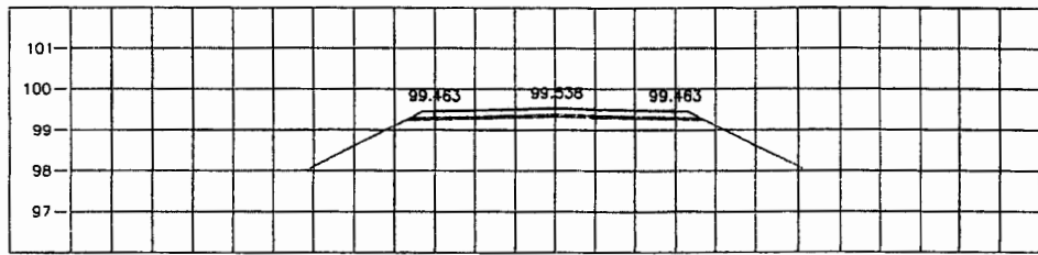
STA. 0+850.000 NGL = 99.327
