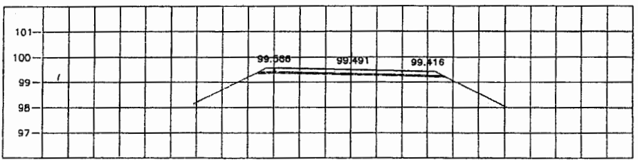
STA. 0+725.000 NGL = 99.156
