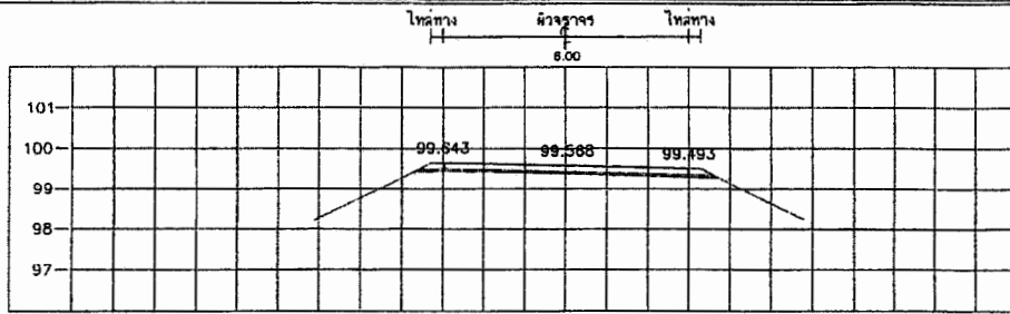
STA. 0+600.000 NGL = 99.249
