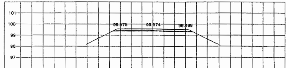
STA. 0+625.000 NGL = 99.339
