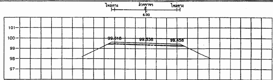
STA. 0+700.000 NGL = 99.317
