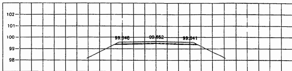
STA. 0+880.000 NGL = 99.652
