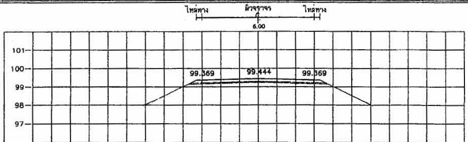
STA. 0+825.000 NGL = 99.202
