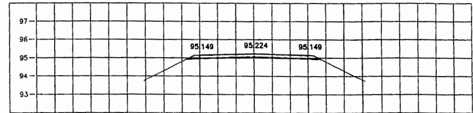
STA. 1+250.000 NGL = 94.962
