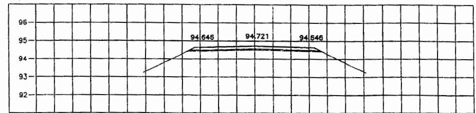
STA. 1+275.000 NGL = 94.369
