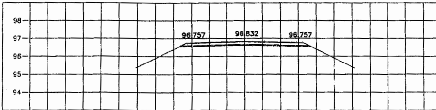
STA. 1+150.000 NGL = 96.440
