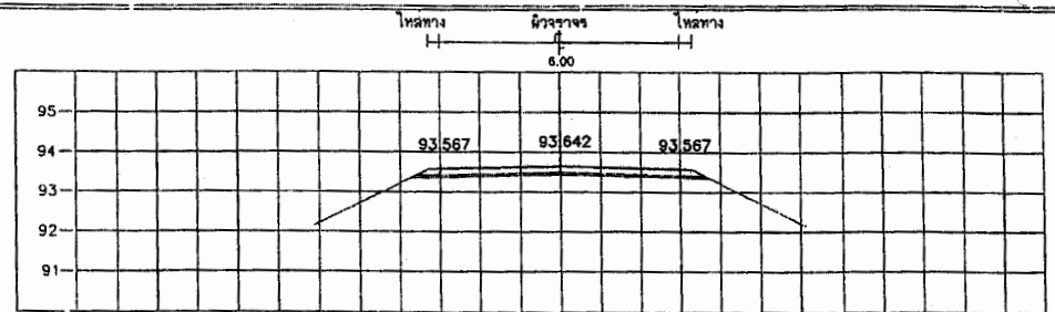
STA. 1+320.000 NGL = 93.342
