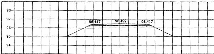
STA. 1+175.000 NGL = 96.050
