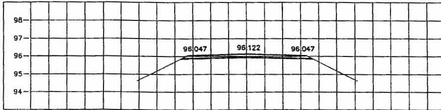
STA. 1+200.000 NGL = 95.732
