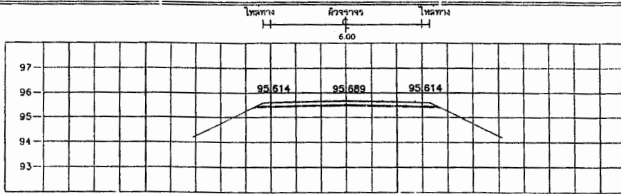
STA. 1+225.000 NGL = 95.395
