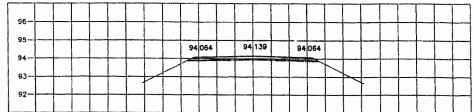
STA. 1+300.000 NGL = 93.762
