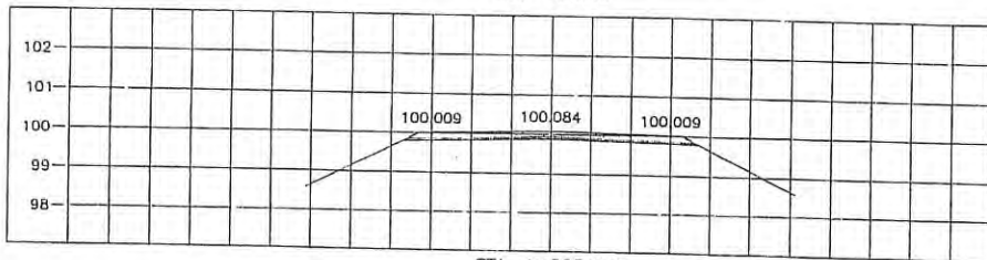
STA. 1+825.000 NGL = 99.779
