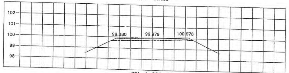
STA. 1+925.000 NGL = 99.709
