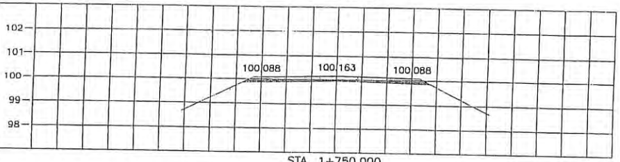
STA. 1+750.000 NGL = 99.958
