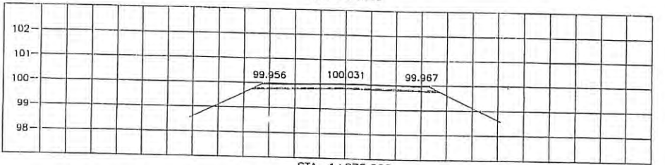
STA. 1+875.000 NGL = 99.770
