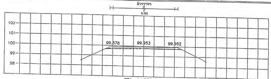
STA. 1+950.000 NGL = 99.682
