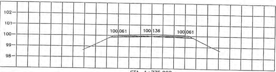
STA. 1+775.000 NGL = 99.853
