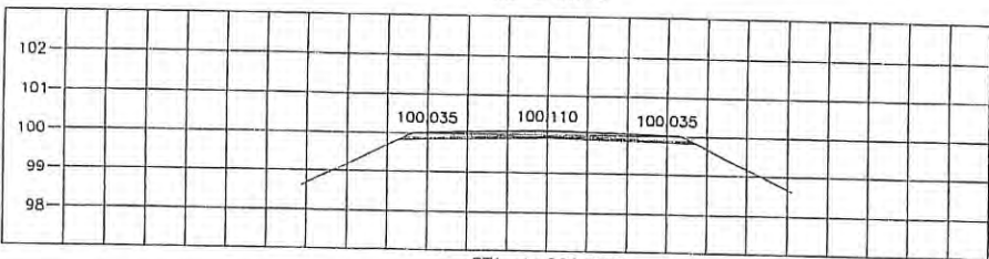
STA. 1+800.000 NGL = 99.832
