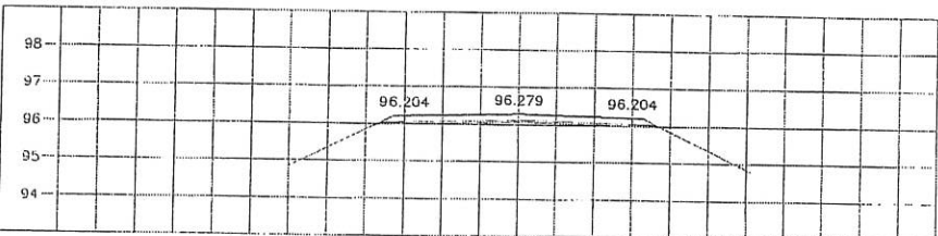
STA. 4+725.000 NGL = 95.917
