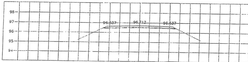
STA. 4+675.000 NGL = 96.344
