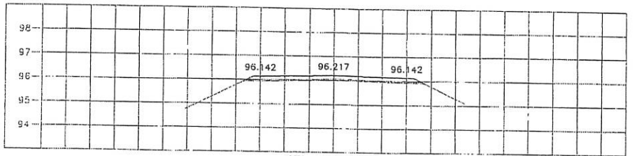
STA. 4+800.000 NGL = 95.917
