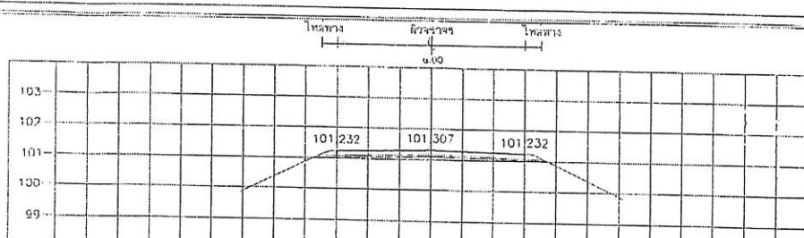
STA. 6+025.000 NGL = 100.833
