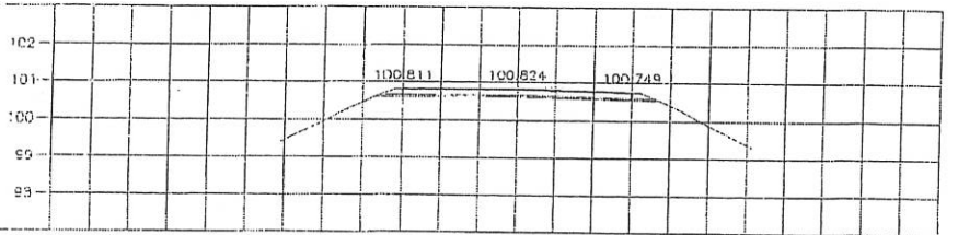
STA. 5+825.000 NGL = 100.428
