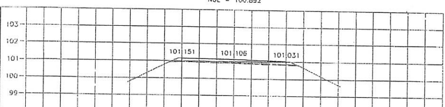
STA. 5+950.000 NGL = 100.814
