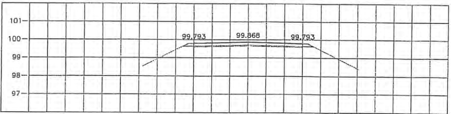
STA. 1+700.000 NGL = 99.471
