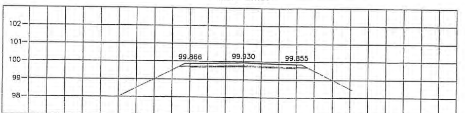
STA. 1+800.000 NGL = 99.614
