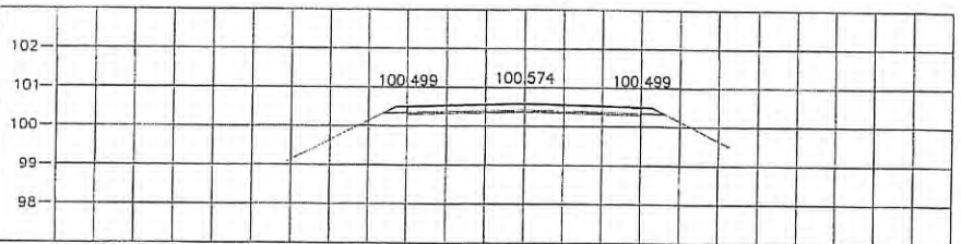
STA. 2+150.000 NGL = 100.392
