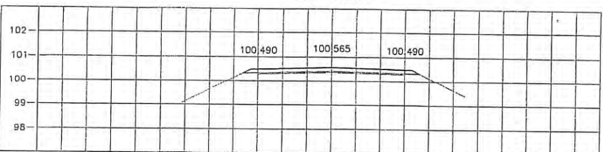
STA. 2+175.000 NGL = 100.404
