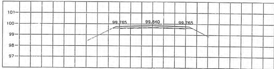
STA. 1+750.000 NGL = 99.495
