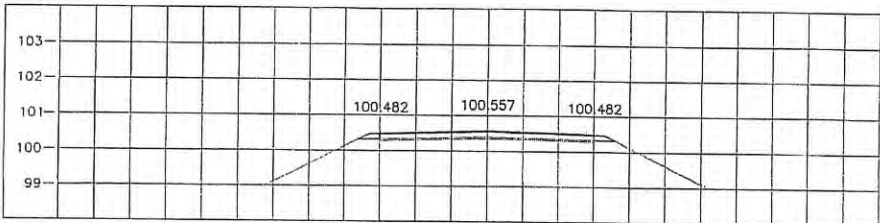
STA. 2+200.000 NGL = 100.523
