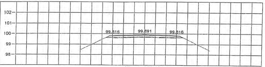
STA. 1+675.000 NGL = 99.525
