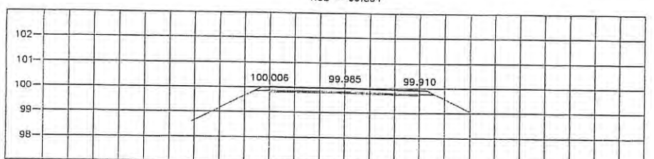
STA. 1+825.000 NGL = 99.734
