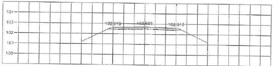
STA. 2+075.000 NGL = 102.323
