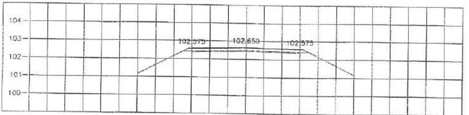
STA. 2+050.000 NGL = 102.289
