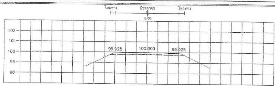
STA. 1+000.000 NGL = 99.706
