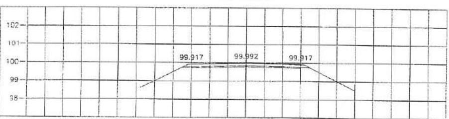
STA. 0+825.000 NGL = 99.768
