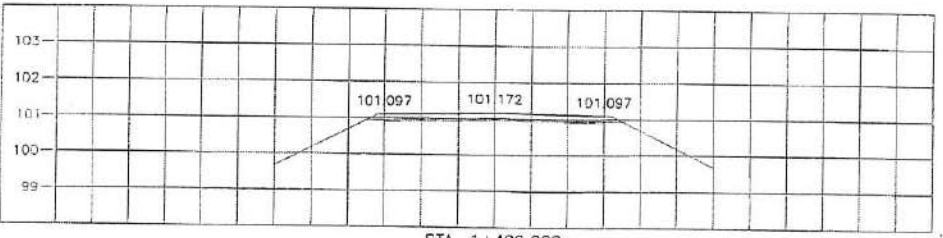
STA. 1+400.000 NGL = 100.762
