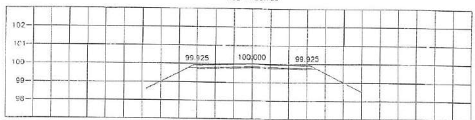
STA. 0+975.000 NGL = 99.637
