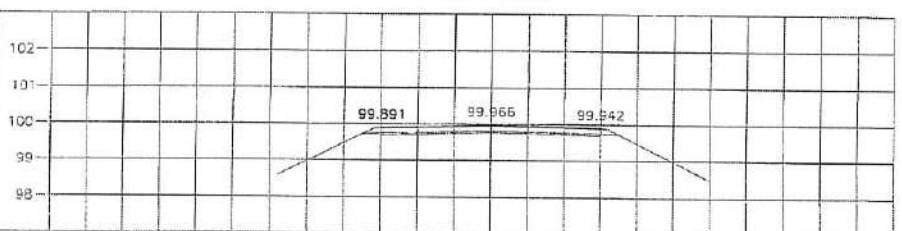
STA. 0+800.000 NGL = 99.965
