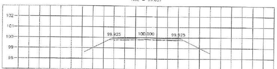
STA. 0+950.000 NGL = 99.627
