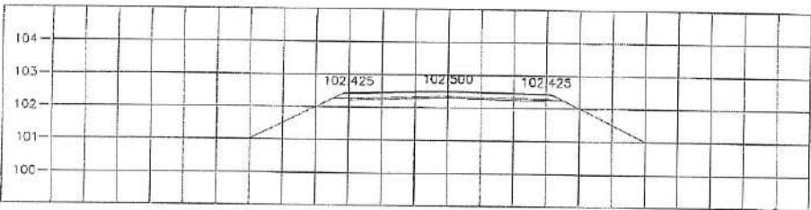
STA. 1+975.000 NGL = 102.149
