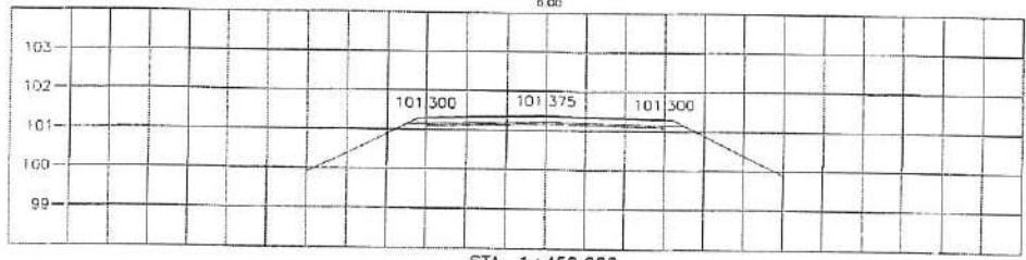
STA. 1+450.000 NGL = 100.950
