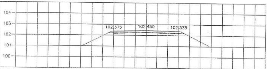
STA. 1+950.000 NGL = 102.061
