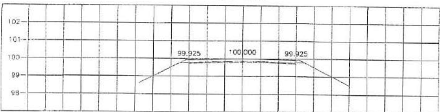
STA. 0+850.000 NGL = 99.719
