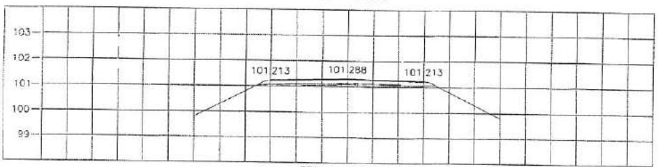
STA. 1+425.000 NGL = 100.826
