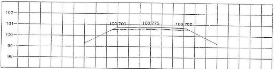
STA. 1+325.000 NGL = 100.277
