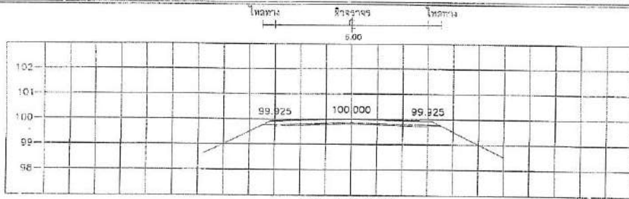
STA. 0+900.000 NGL = 99.752
