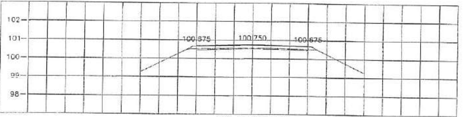
STA. 1+300.000 NGL = 100.366
