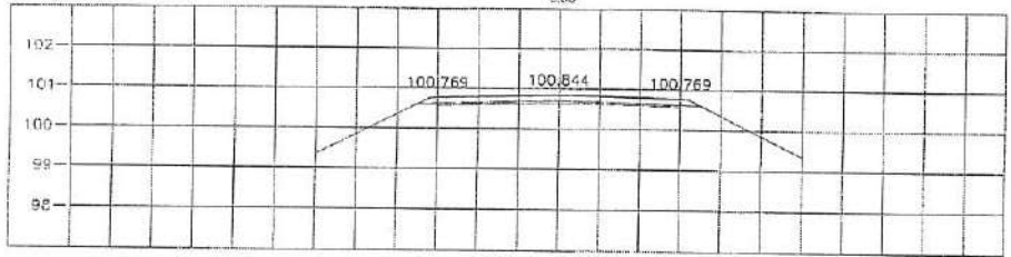
STA. 1+350.000 NGL = 100.348
