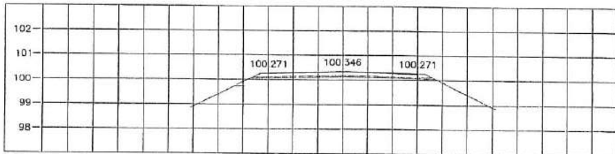
STA. 1+100.000 NCL = 100.066
