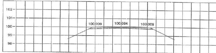
STA. 1+825.000 NGL = 99.779
