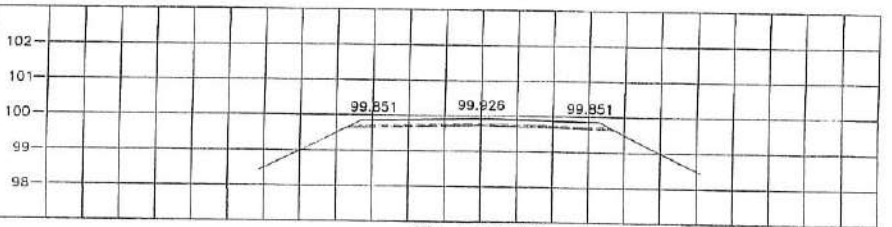
STA. 1+975.000 NGL = 99.767
