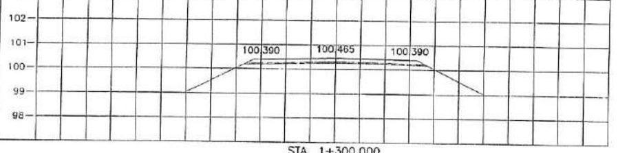
STA. 1+300.000 NCL = 100.190
