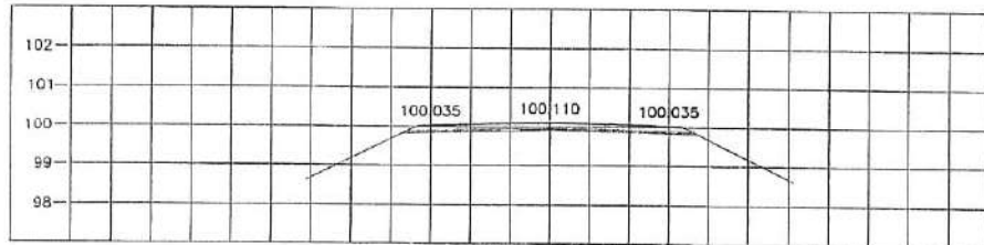
STA. 1+800.000 NGL = 99.832
