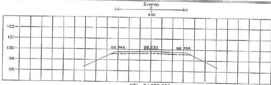
STA. 2+075.000 NGL = 99.640
