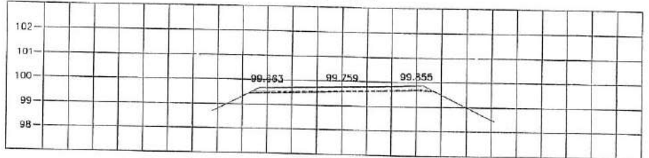
STA. 2+150.000 NGL = 99.649
