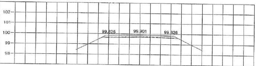
STA. 2+000.000 NGL = 99.727
