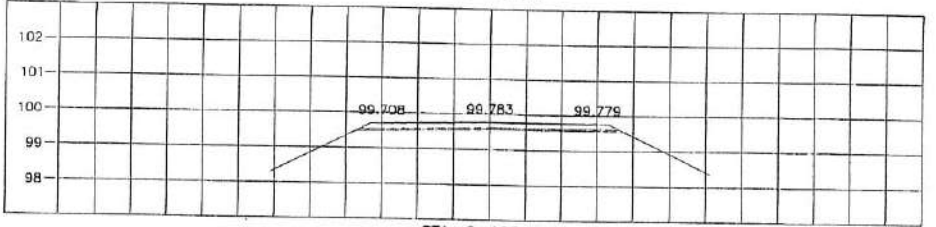
STA. 2+125.000 NGL = 99.599
