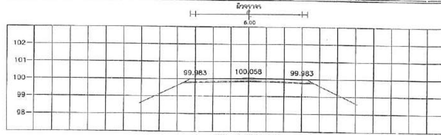
STA. 1+850.000 NGL = 99.743
