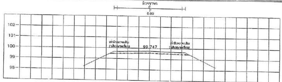
STA. 2+163.000 NGL = 99.747
