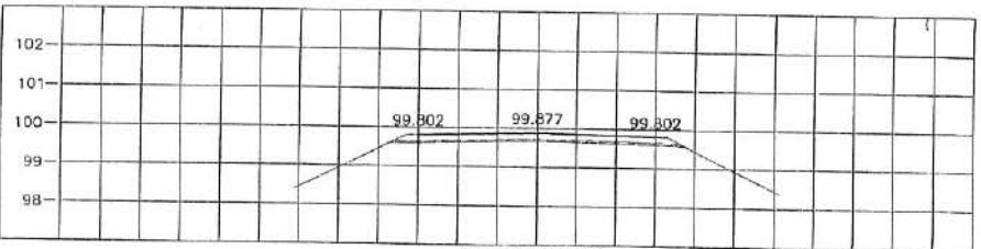
STA. 2+025.000 NGL = 99.684
