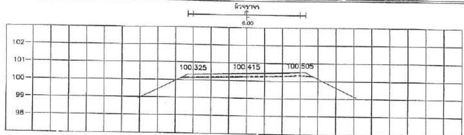
STA. 1+500.000 NCL = 100.031
