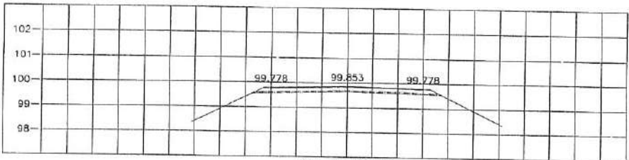
STA. 2+050.000 NGL = 99.669
