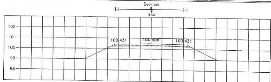
STA. 1+400.000 NCL = 100.309
