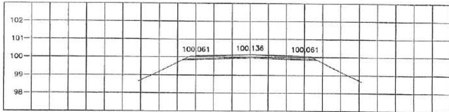
STA. 1+775.000 NGL = 99.853
