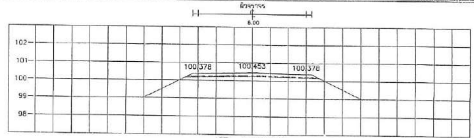
STA. 1+275.000 NCL = 100.138
