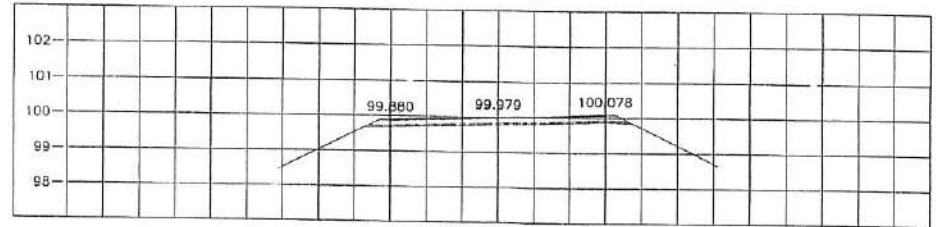
STA. 1+925.000 NGL = 99.709
