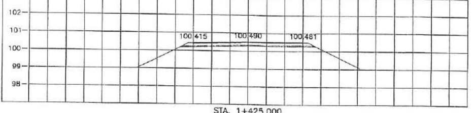
STA. 1+425.000 NCL = 100.277
