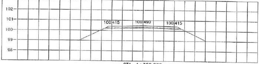
STA. 1+350.000 NCL = 100.240
