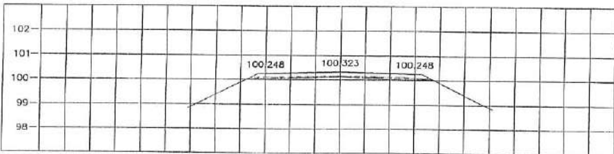
STA. 1+075.000 NCL = 100.036
