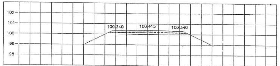
STA. 1+200.000 NCL = 100.144
