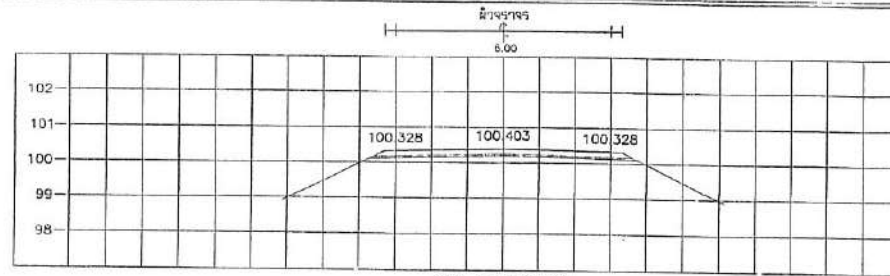
STA. 1+175.000 NCL = 100.073
