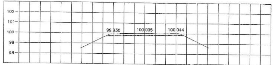
STA. 1+900.000 NGL = 99.768
