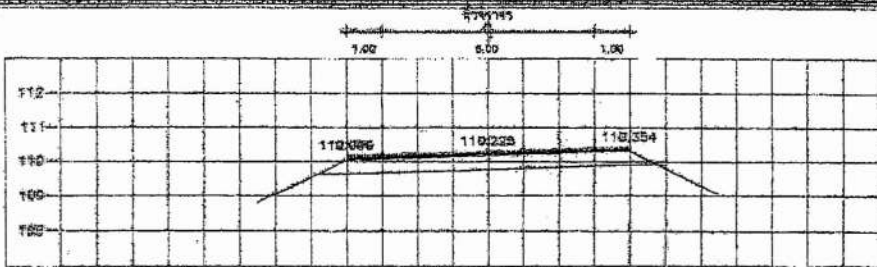
STA. 6+668.000 NGL = 110.088
