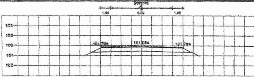
STA 5+500.000 NGL = 101.890
