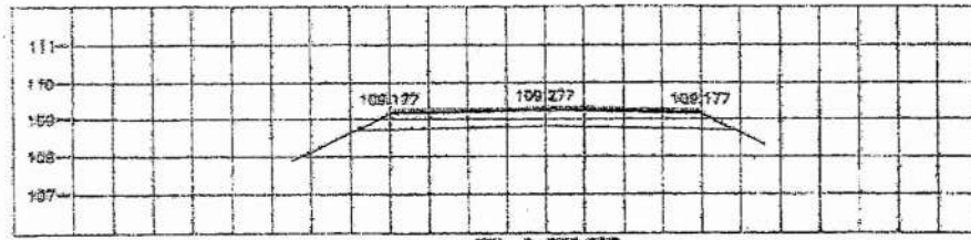
STA. 6+750.000 NGL = 109.233
