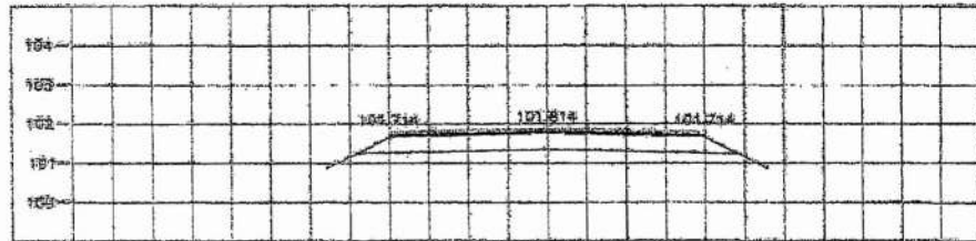
STA. 5+305.000 NGL = 101.736
