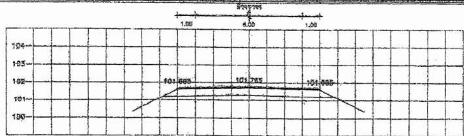
STA. 5+375.000 NGL = 101.590
