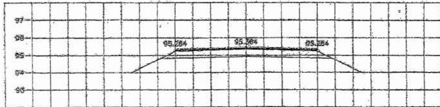
STA. 4+558.000 NCL = 95.184
