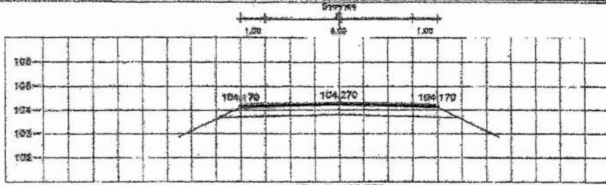
STA. 5+400.000 NGL = 104.082
