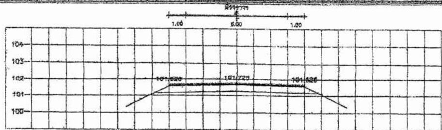
STA 5+800.000 NGL = 101.626
