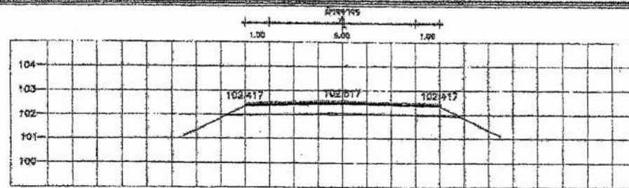
STA. 6+275.000 NGL = 102.371
