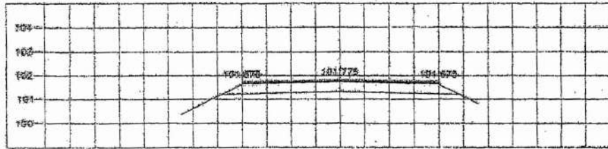
STA 5+450.000 NGL = 101.678
