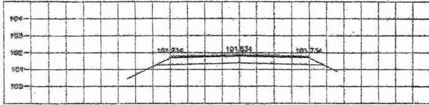
STA 5+475.000 NGL = 101.731
