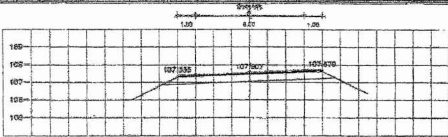
STA 8+625.000 NGL = 107.371
