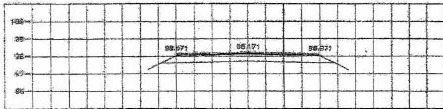
STA. 4+325.000 NGL = 98.099
