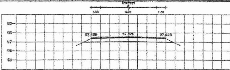
STA. 4+373.000 NGL = 97.489
