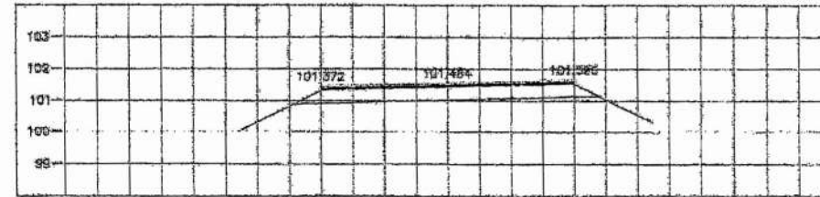
STA. 6+200.000 NGL = 101.393
