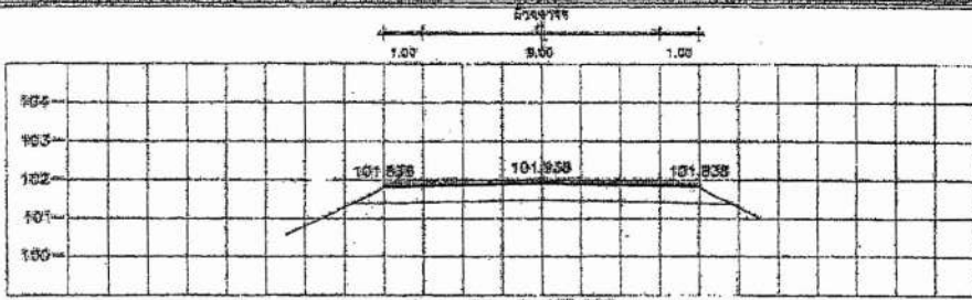
STA. 5+275.000 NGL = 101.828
