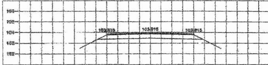
STA. 5+375.000 NGL = 103.699
