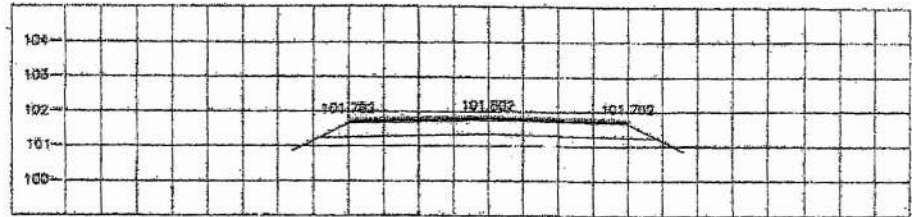
STA 5+875.000 NGL = 101.716
