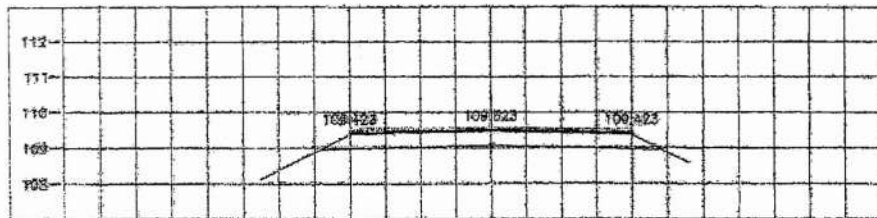
STA. 6+725.000 NGL = 109.510
