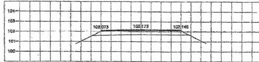
STA. 6+265.000 NGL = 102.033
