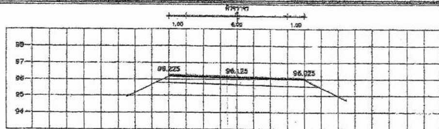
STA. 4+475.000 NGL = 96.072
