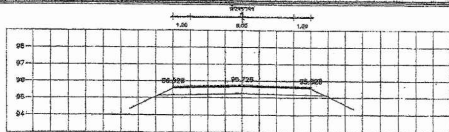
STA. 4+700.000 NCL = 95.541
