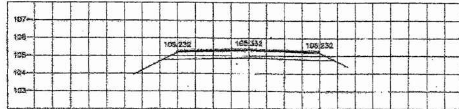
STA. 5+475.000 NGL = 105.202
