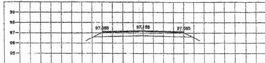
STA. 4+406.000 NGL = 97.133
