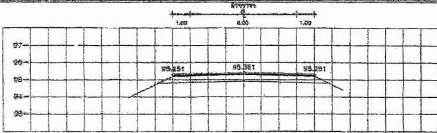
STA. 4+600.000 NCL = 95.212
