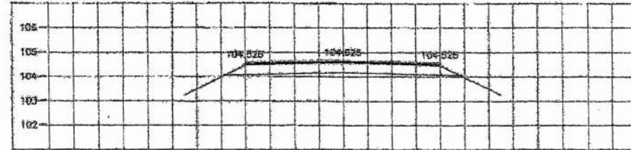
STA. 5+425.000 NGL = 104.461
