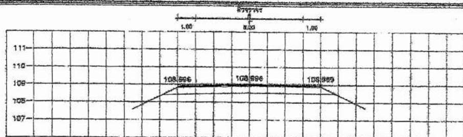
STA 8+725.000 NGL = 106.880
