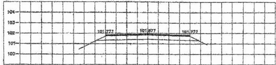
STA 5+850.000 NGL = 101.794
