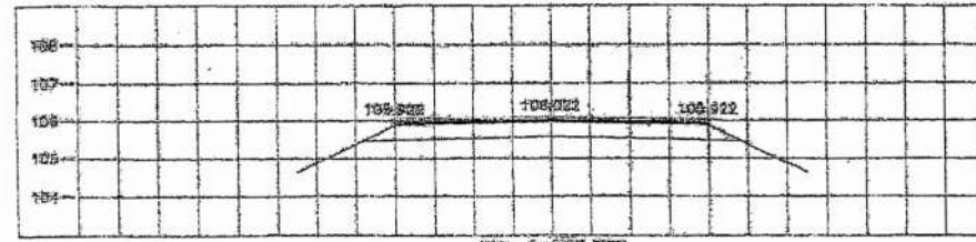
STA 8+525.000 NGL = 106.888
