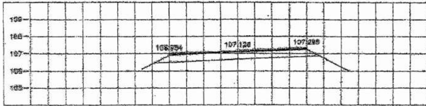
STA 8+600.000 NGL = 106.976
