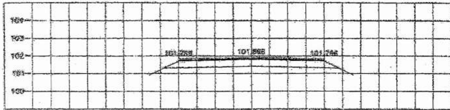
STA. 5+295.000 NGL = 101.793
