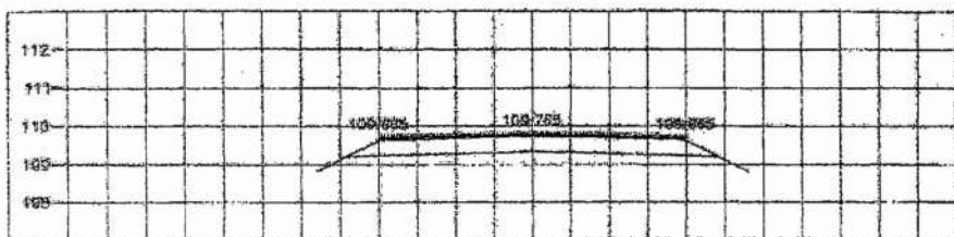
STA. 6+696.000 NGL = 109.737
