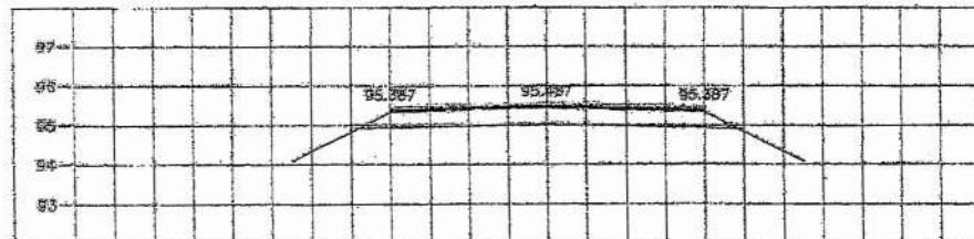
STA. 4+525.000 NCL = 95.320
