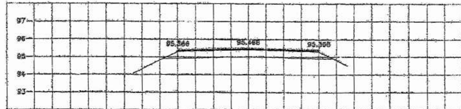
STA. 4+680.000 NCL = 95.354
