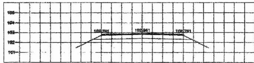
STA. 6+308.000 NGL = 102.751
