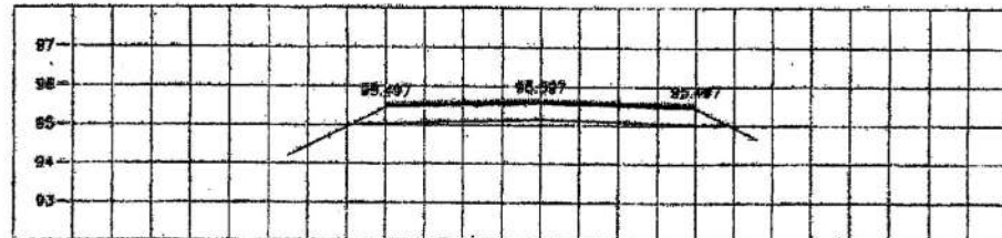
STA 4+675.000 NGL = 95.485
