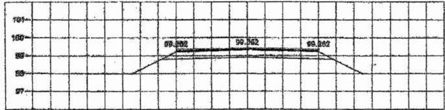
STA 4+975.000 NGL = 99.330
