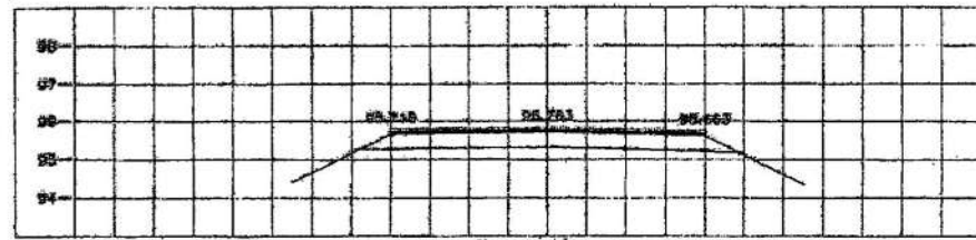
STA 4+608.000 NGL = 95.638
