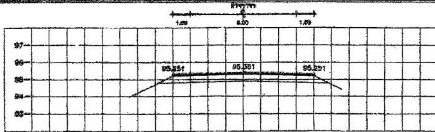
STA 4+603.000 NGL = 95.212
