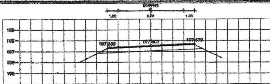
STA. 6+625.000 NGL = 107.371
