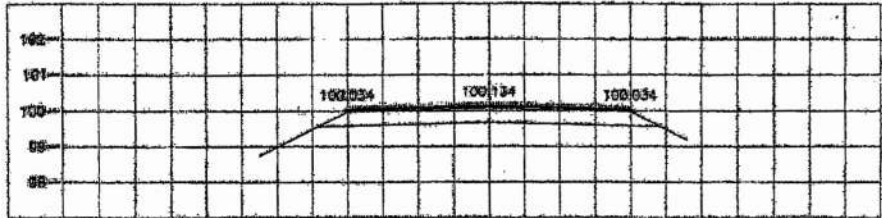
STA 5+025.000 NGL = 100.642
