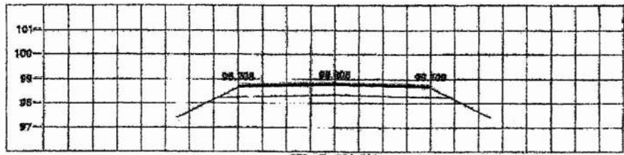
STA 5+800.000 NGL = 98.554
