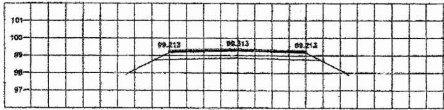
STA 5+750.000 NGL = 98.155
