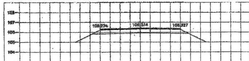
STA. 6+650.000 NGL = 108.231
