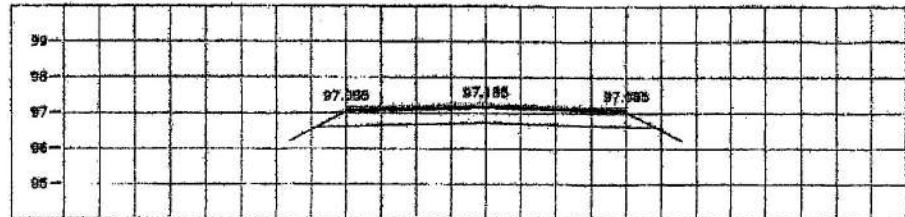
STA. 4+400.000 NGL = 97.133
