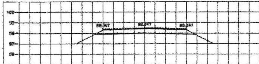
STA. 4+360.000 NGL = 96.324
