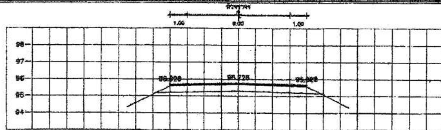
STA 4+700.000 NGL = 95.541
