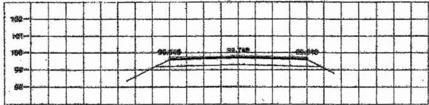
STA 5+000.000 NGL = 99.678
