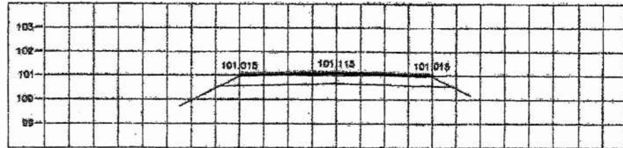
STA 5+100.000 NGL = 101.020
