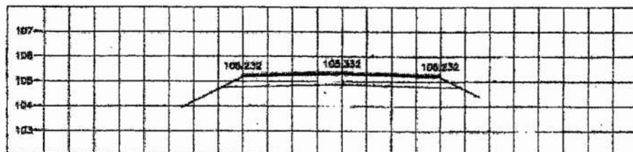
STA. 6+475.000 NGL = 105.202
