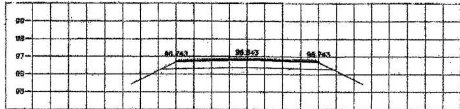
STA. 4+425.000 NGL = 96.719
