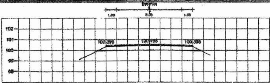
STA 5+050.000 NGL = 100.430
