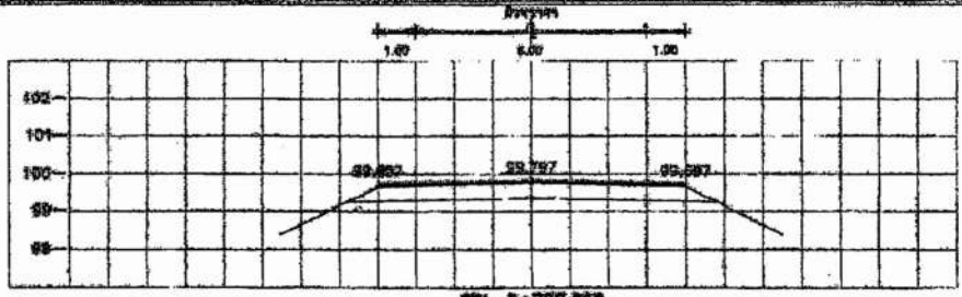
STA 5+725.000 NGL = 99.912
