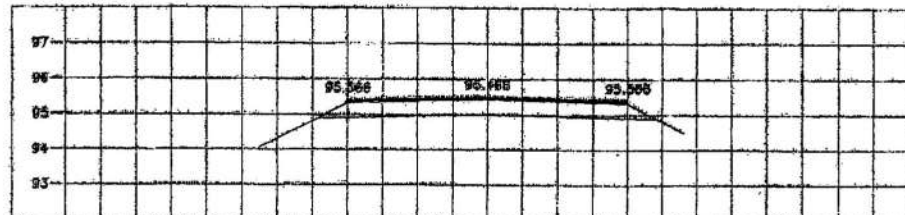
STA 4+680.000 NGL = 95.354
