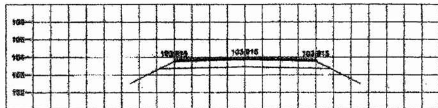
STA. 6+375.000 NGL = 103.899
